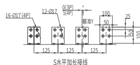
S水平加长接线
