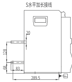
连接尺寸
