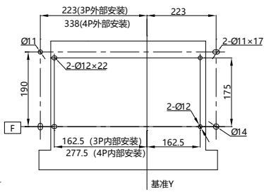
安装尺寸
