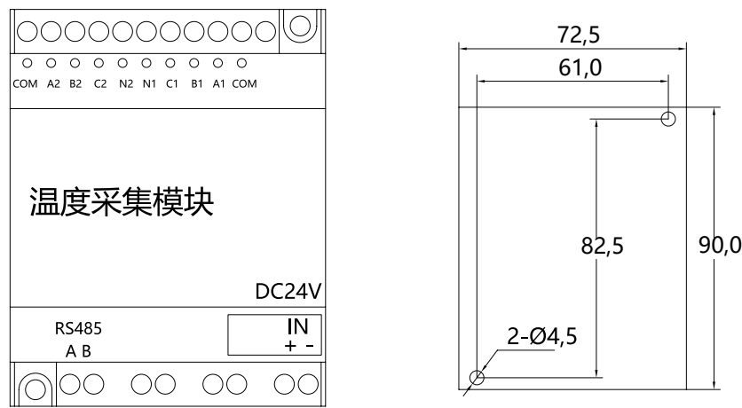
无线温度监测单元（导轨型）外形及安装尺寸
