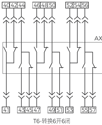
T6-转换6开6闭
