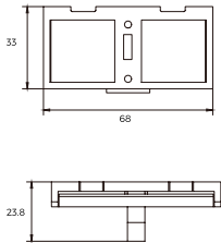
1600 壳架外形尺寸
