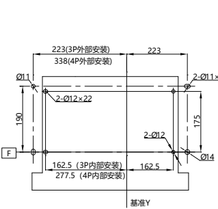
安装尺寸
