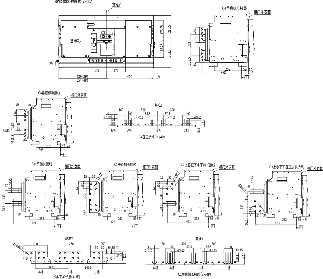
BW3-8000抽屉式(7500A)
