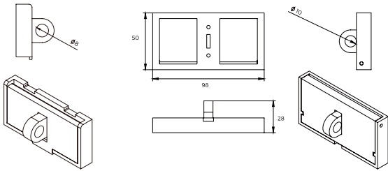
2000 壳架及以上外形尺寸
