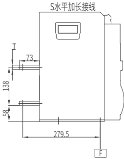
安装尺寸
