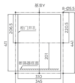
面板开孔尺寸
