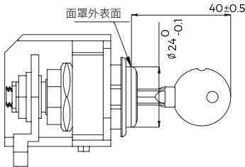
2000 壳架及以上钥匙锁外形尺寸
