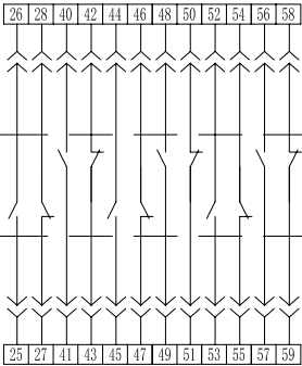
D6-独立6开6闭(2500壳架)
