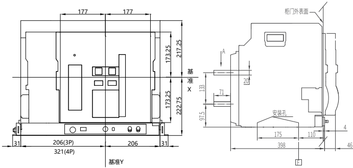
外形尺寸
