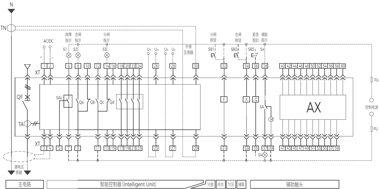
BW3-2500/3200/4000/5000/6300/8000 二次回路接线图
