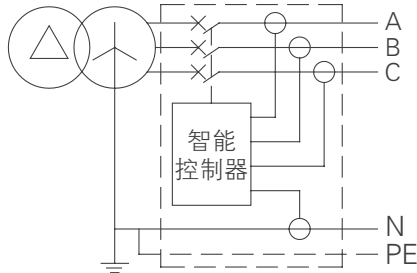
3P+N 例 TN-S 系统
