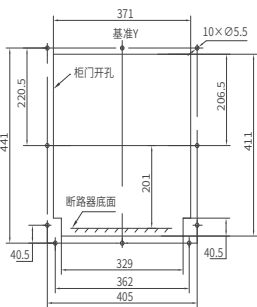
面板开孔尺寸
