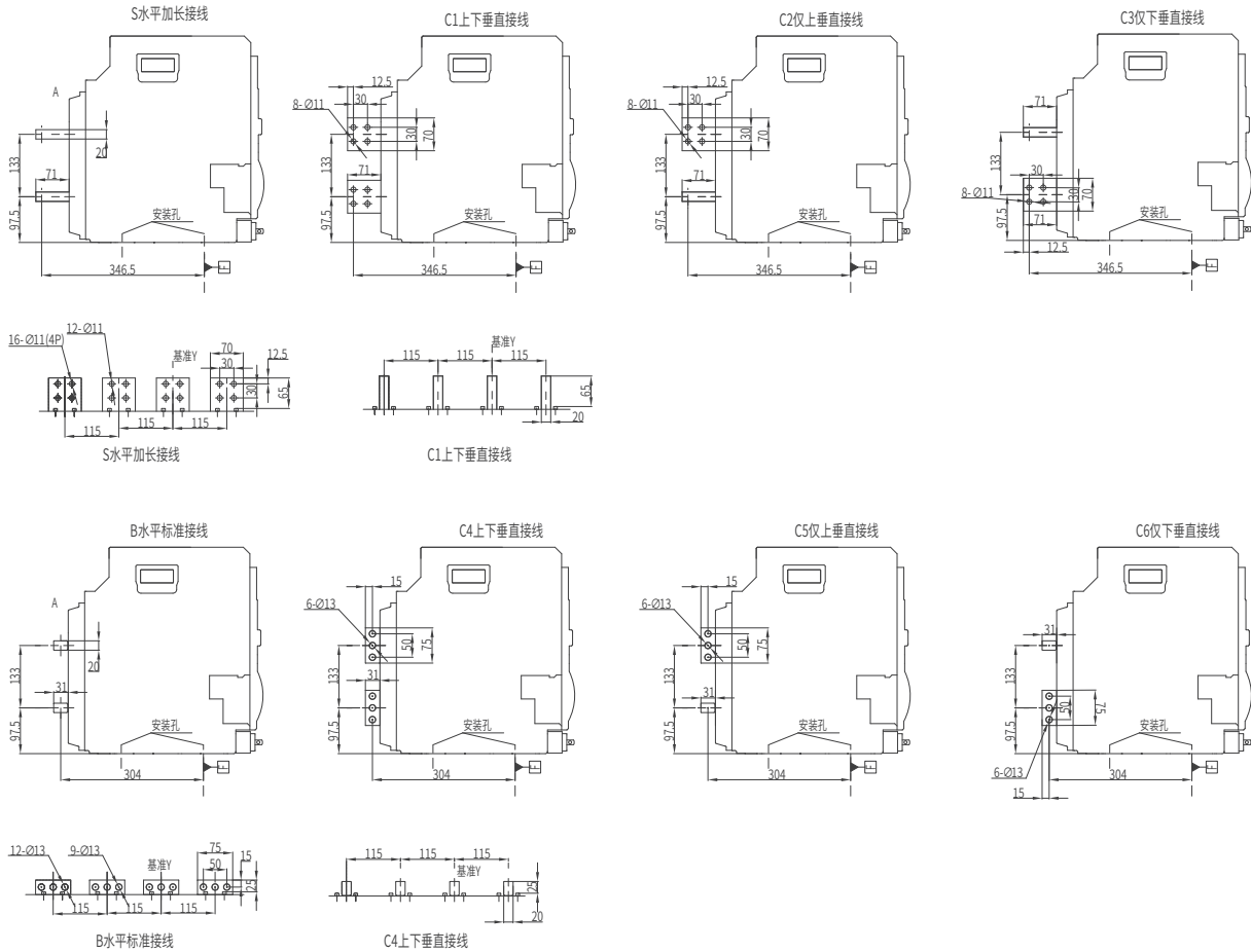
连接尺寸
