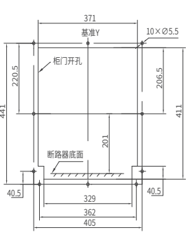
面板开孔尺寸
