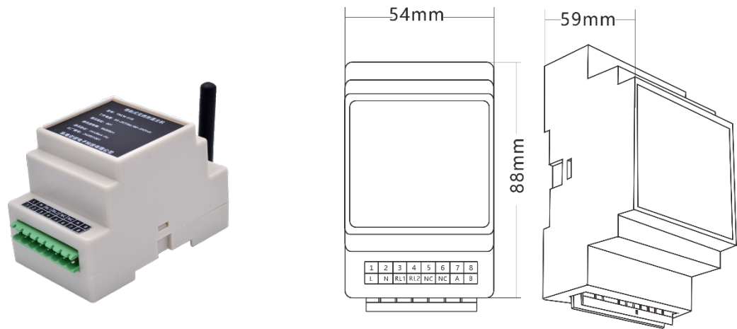
无线温度监测单元（导轨型）外形及安装尺寸
