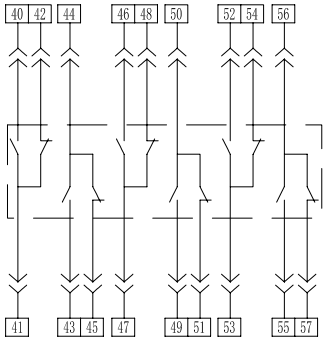
T6-转换6开6闭
