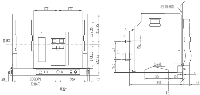
外形尺寸
