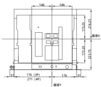
连接尺寸
