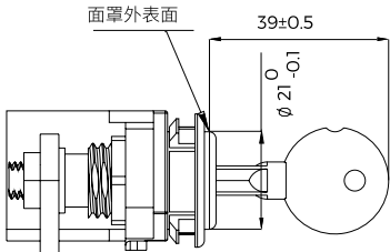
1600 壳架钥匙锁外形尺寸
