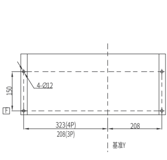
安装尺寸
