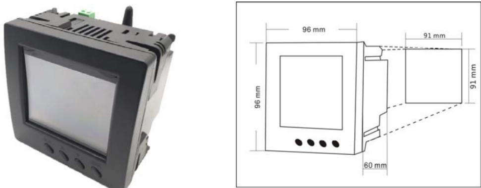
有线温度传感器安装尺寸
