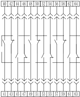
D6-独立6开6闭(3200壳架及以上)
