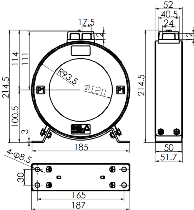
图 25-2 ZT120 互感器
