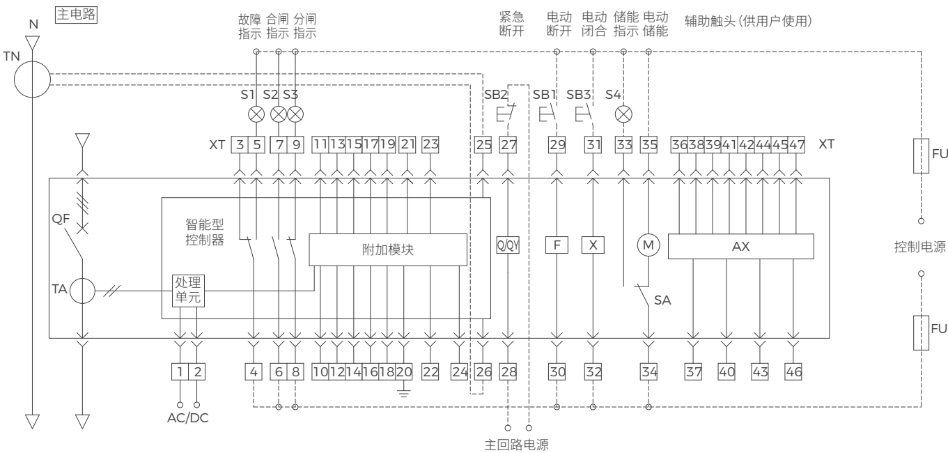
工作原理图 BW1-1600 的二次接线图
