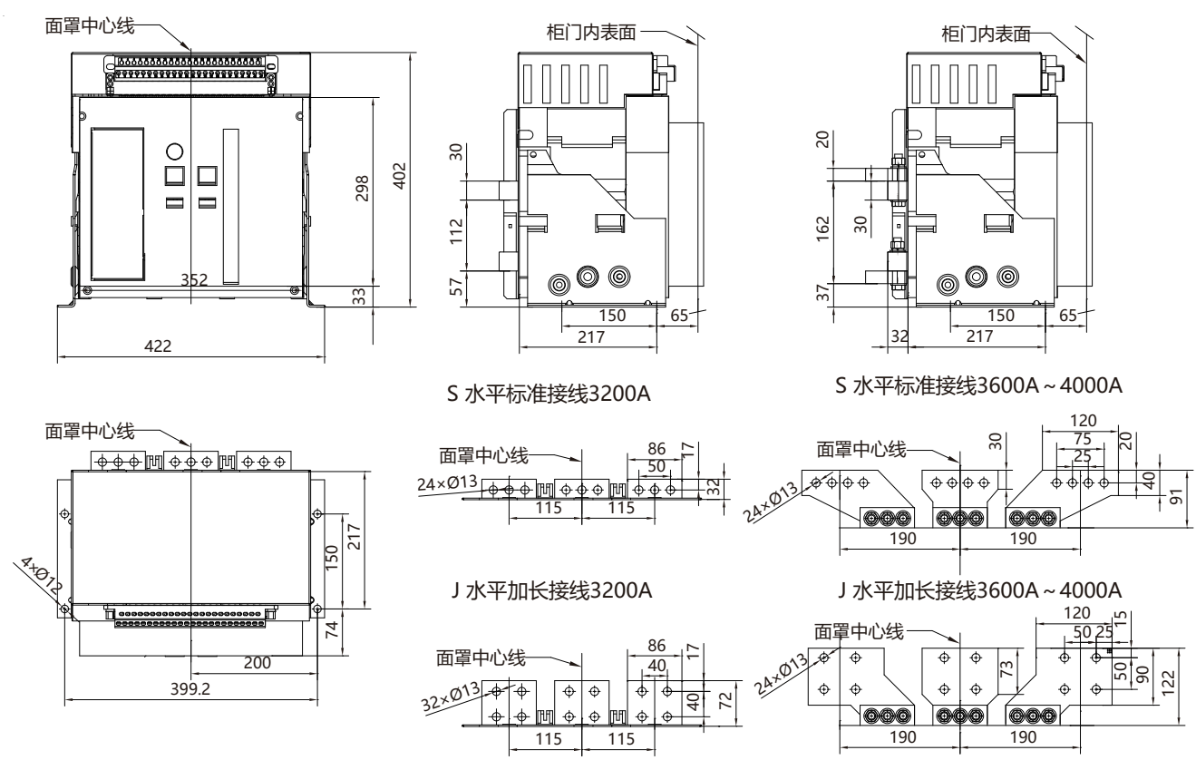
图 40 固定式断路器安装尺寸及外形尺寸 (BW1-4000/3)
