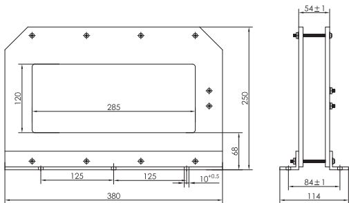
图 26-1 BH-0.66-285×120 互感器
