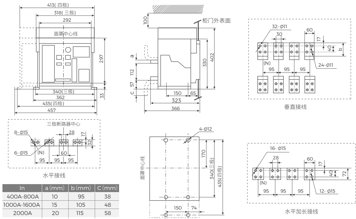
固定式断路器安装尺寸及外形尺寸
