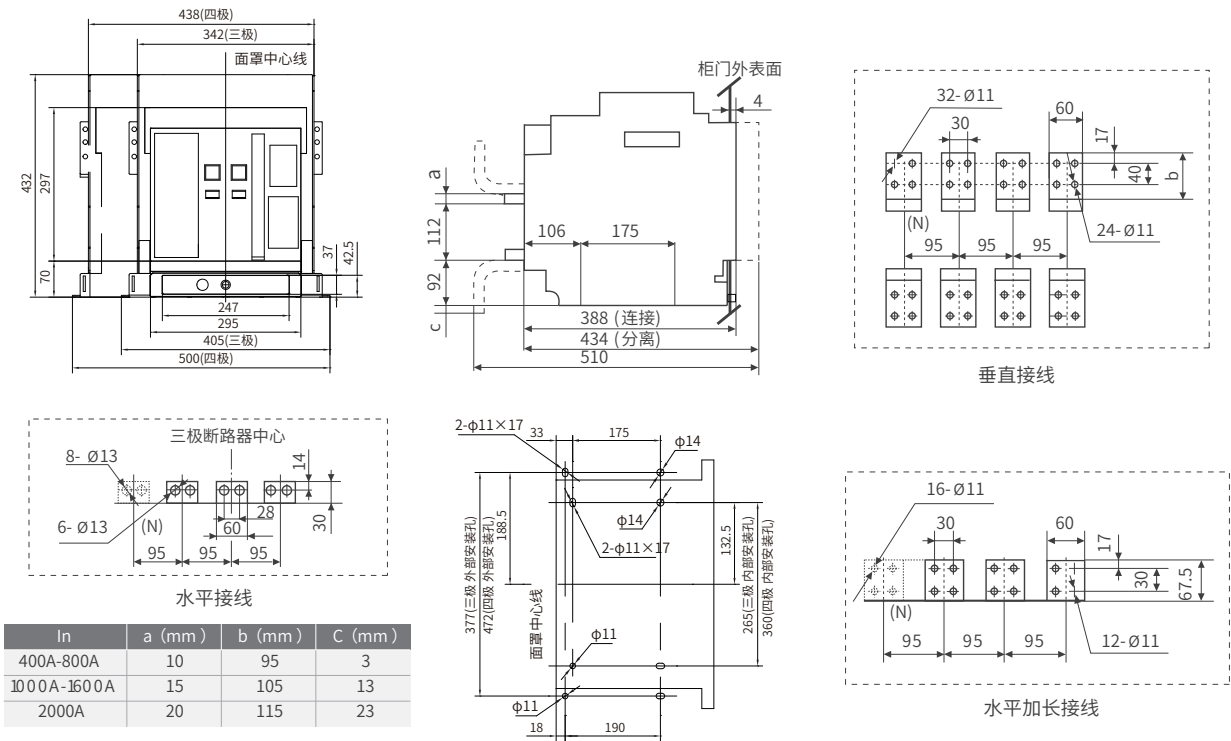
图 44 抽屉式断路器安装尺寸及外形尺寸 (BW1-2000)
