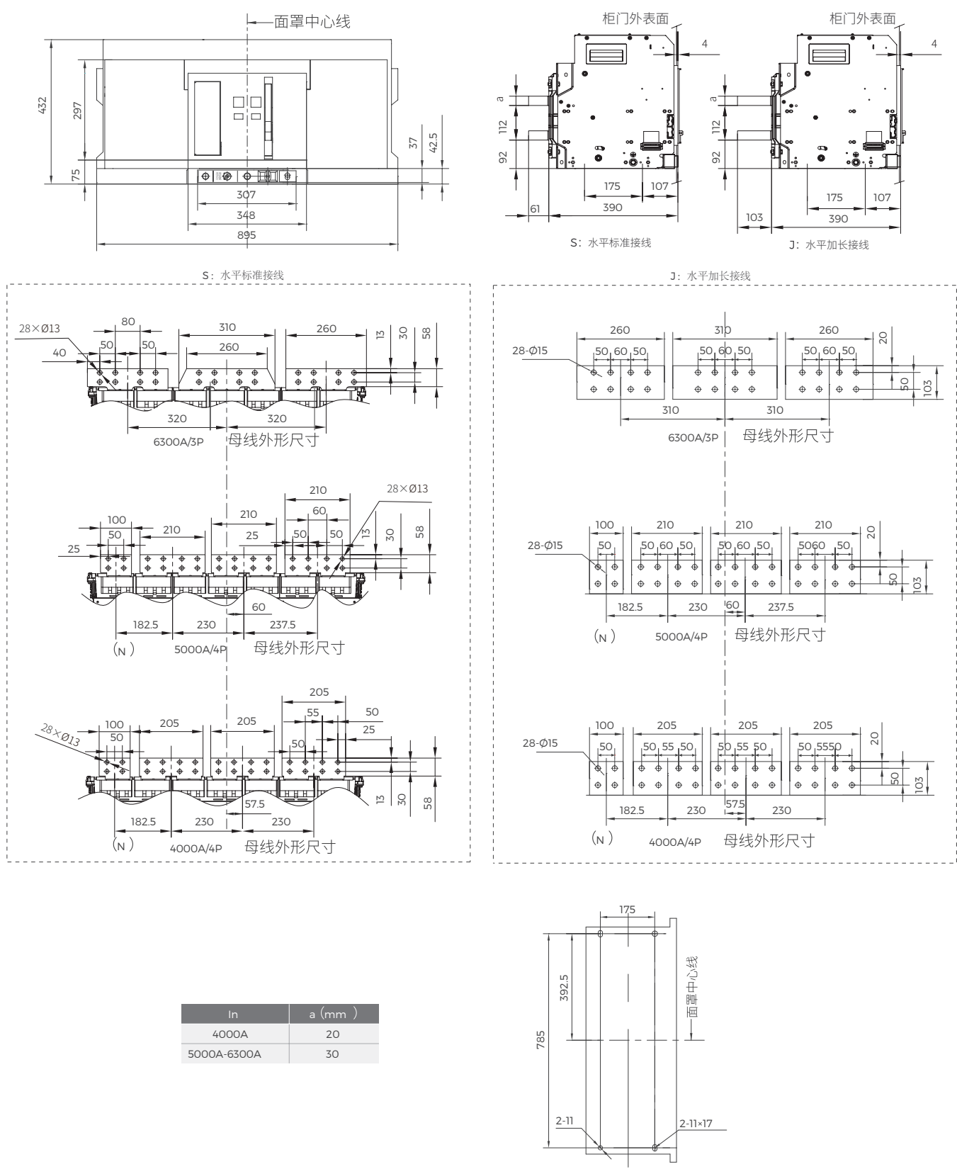
图 49 抽屉式断路器安装尺寸及外形尺寸 ( BW1-6300 4000/4P、BW1-6300 5000/4P)、BW1-6300 6300/3P )
