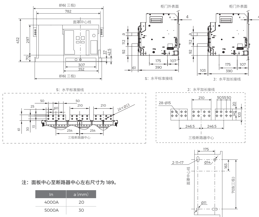
图 48 抽屉式断路器安装尺寸及外形尺寸 (BW1-6300 4000/3P、BW1-6300 5000/3P)
