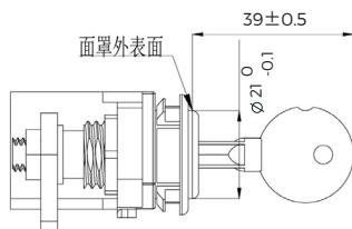
图 27-1 1600A 壳架开孔尺寸
