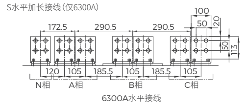
S水平加长接线 (仅6300A)
