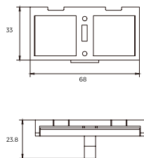
1600 壳架外形尺寸
