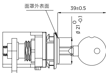
1600 壳架钥匙锁外形尺寸
