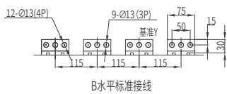
B水平标准接线
