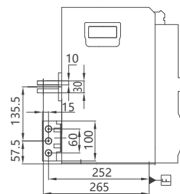
C6仅下垂直接线 (4000A ~ 5000A)
