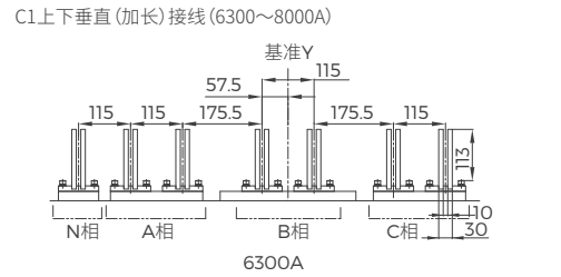
C1上下垂直 (加长) 接线 (6300~8000A)
