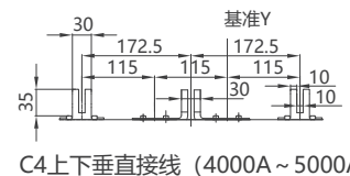
C4上下垂直接线 (4000A ~ 5000A)
