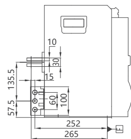
C6仅下垂直接线 (4000A ~ 5000A)
