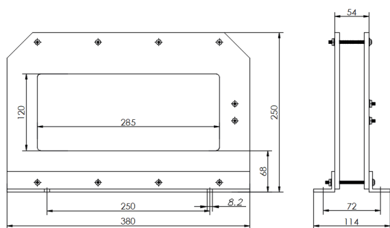
图 26-1 BH-LMB-280×120 互感器
