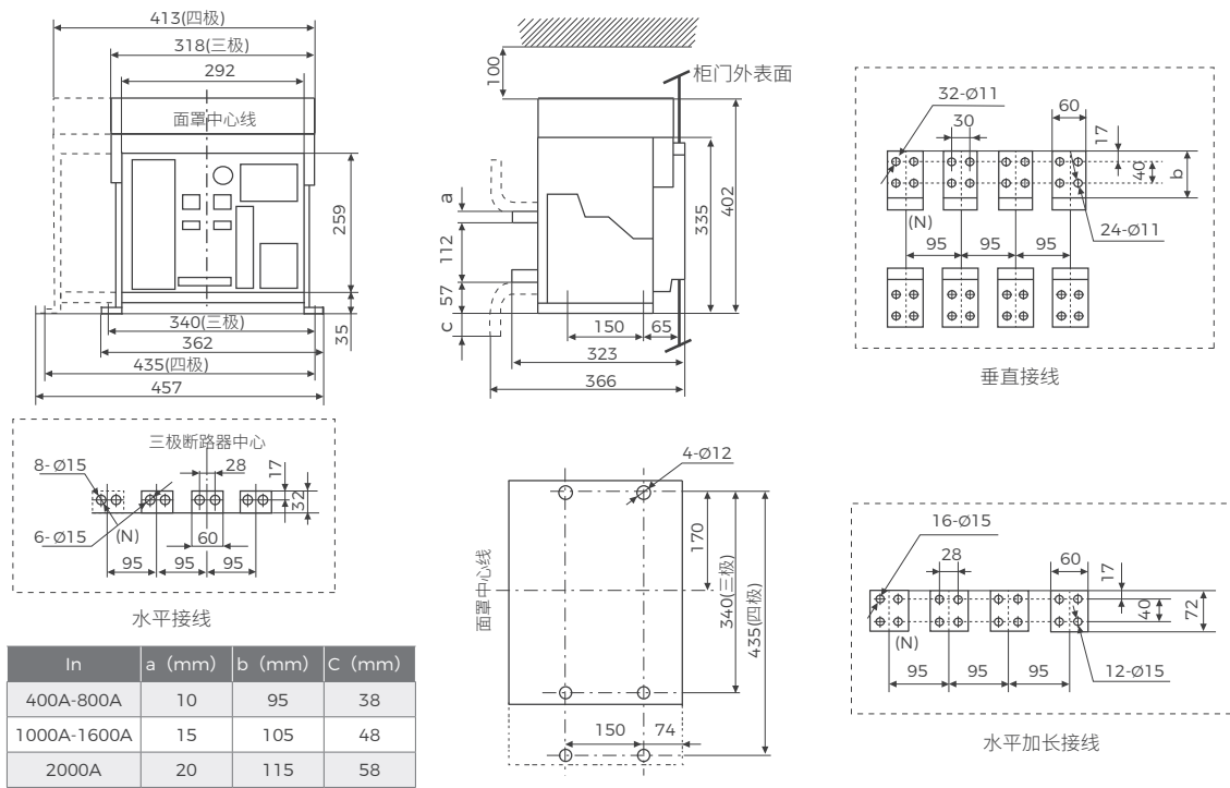
图 38 固定式断路器安装尺寸及外形尺寸 (BW1A-2000)
