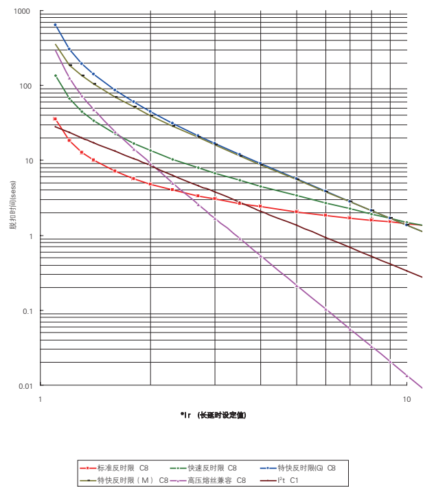
不同曲线类型对比（曲线速率：C8）
