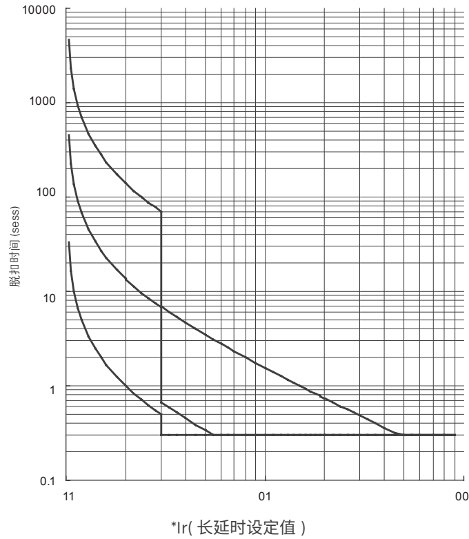
反时限保护示例
