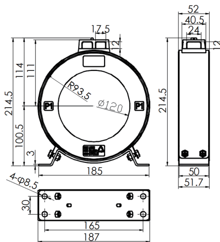
图 25-2 ZT120 互感器
