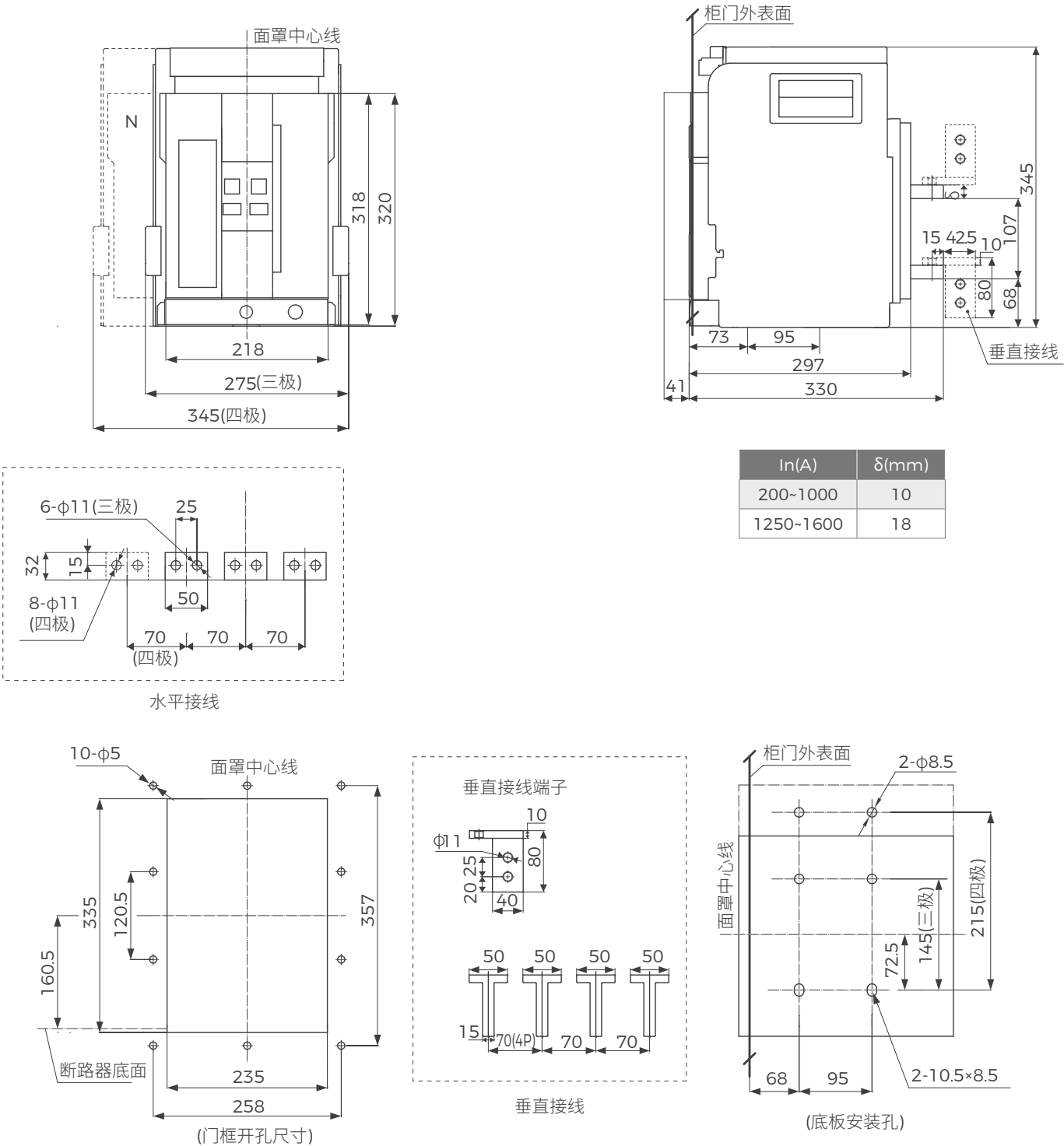
图 43 抽屉式断路器安装尺寸及外形尺寸 (BW1A-1600)
