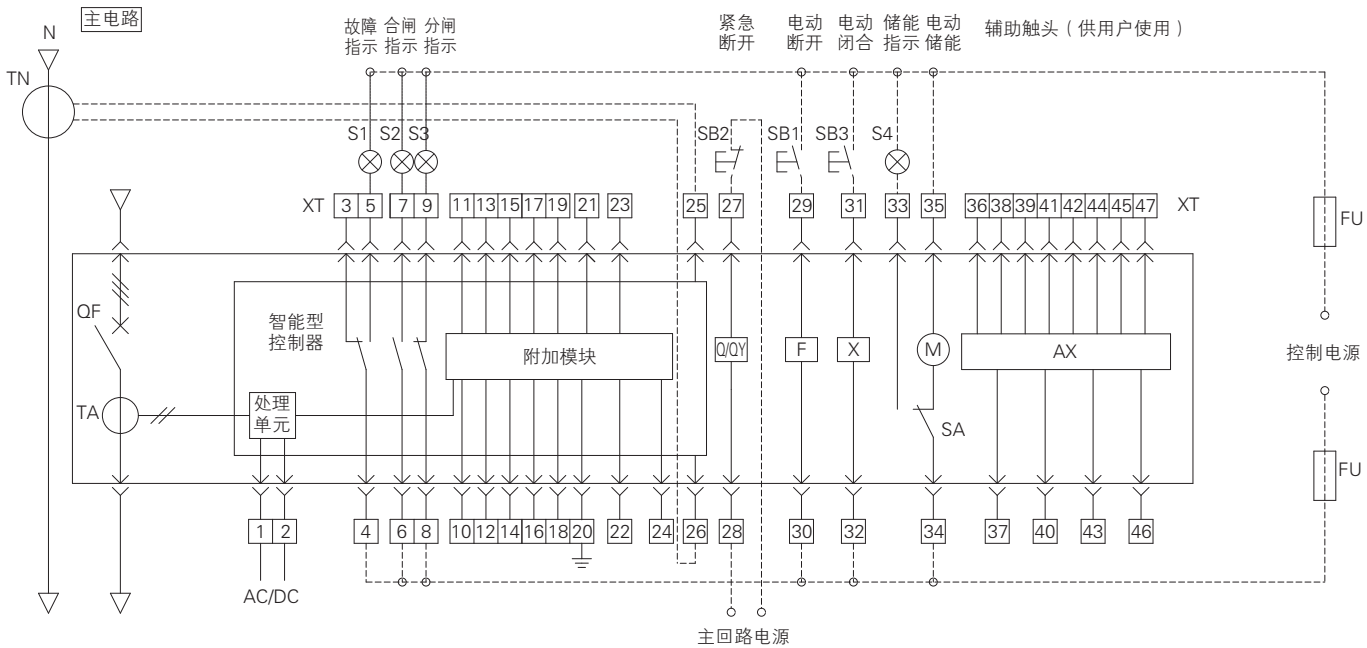
工作原理图 BW1A-1600 的二次接线图
