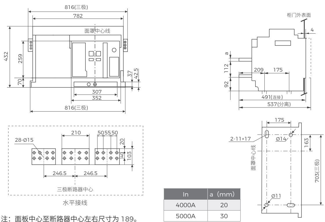
图 48 抽屉式断路器安装尺寸及外形尺寸 (BW1A-6300 4000/3P、BW1A-6300 5000/3P)
