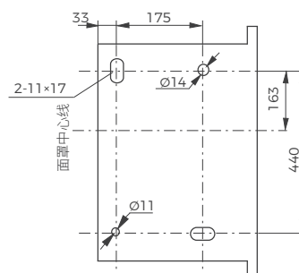
图 46 抽屉式断路器安装尺寸及外形尺寸 (BW1A-4000/3)
