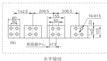
图 47 抽屉式断路器安装尺寸及外形尺寸 (BW1A-4000/4)
