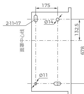
图 47 抽屉式断路器安装尺寸及外形尺寸 (BW1A-4000/4)
