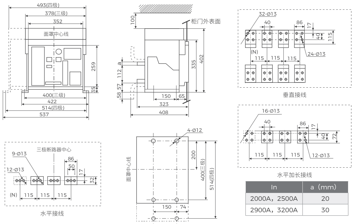
图 39 固定式断路器安装尺寸及外形尺寸 (BW1A-3200)
