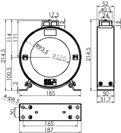
图 25-2 ZT120 互感器
