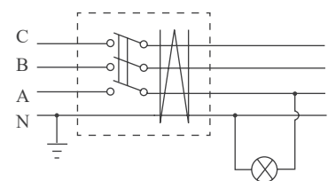
正确接线
