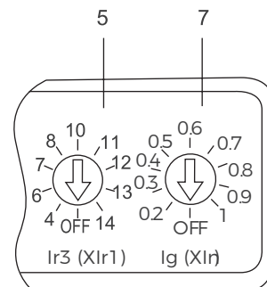
BM3E-800, In=800A 电子式脱扣器 (C型接地保护)
