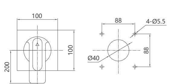
1600 壳架“F”型手柄外形及门板开孔尺寸
