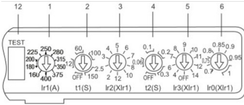
BM3E-400, In=400A 电子式脱扣器
