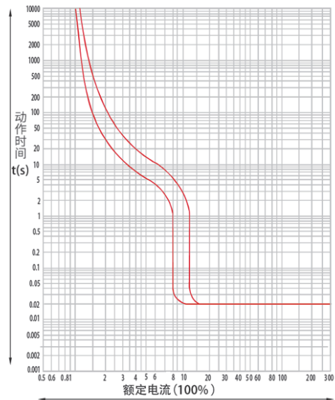
时间/特性曲线
