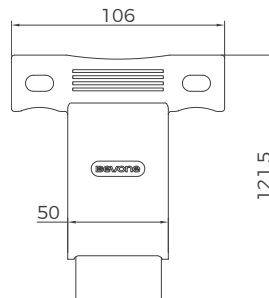
加长手柄外形尺寸图
