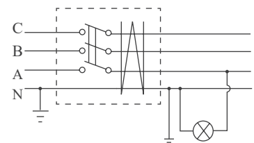
错误接线
