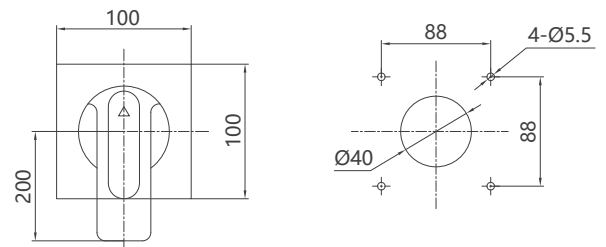
1600 壳架 “F”型手柄外形及门板开孔尺寸
