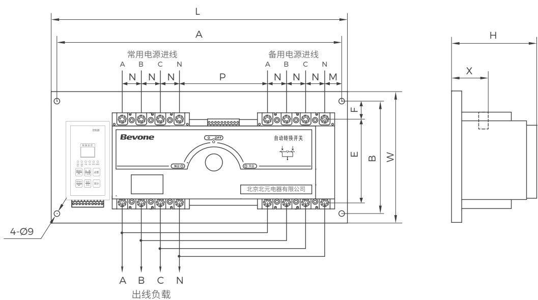
BM30Q1-125、250/4P 外形、安装尺寸及接线图
