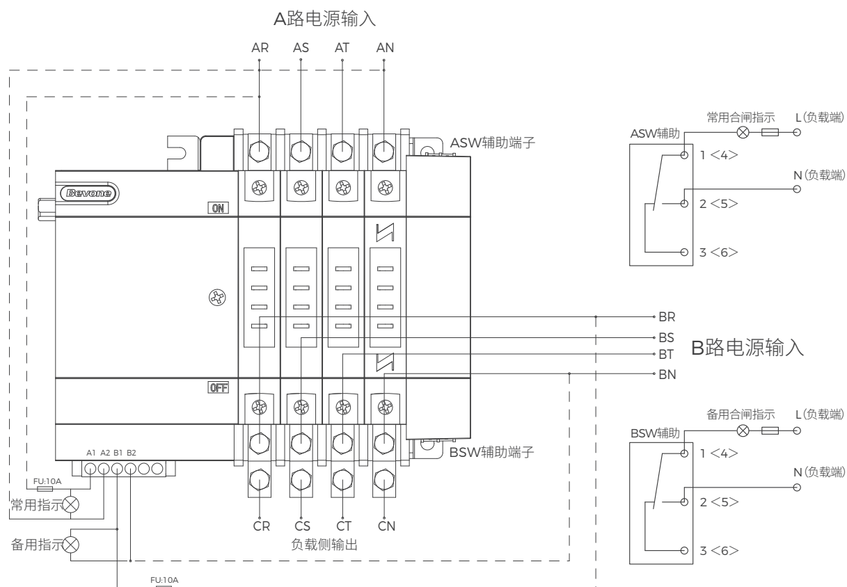
BQ3-80A~5000A N 型控制器接线图
