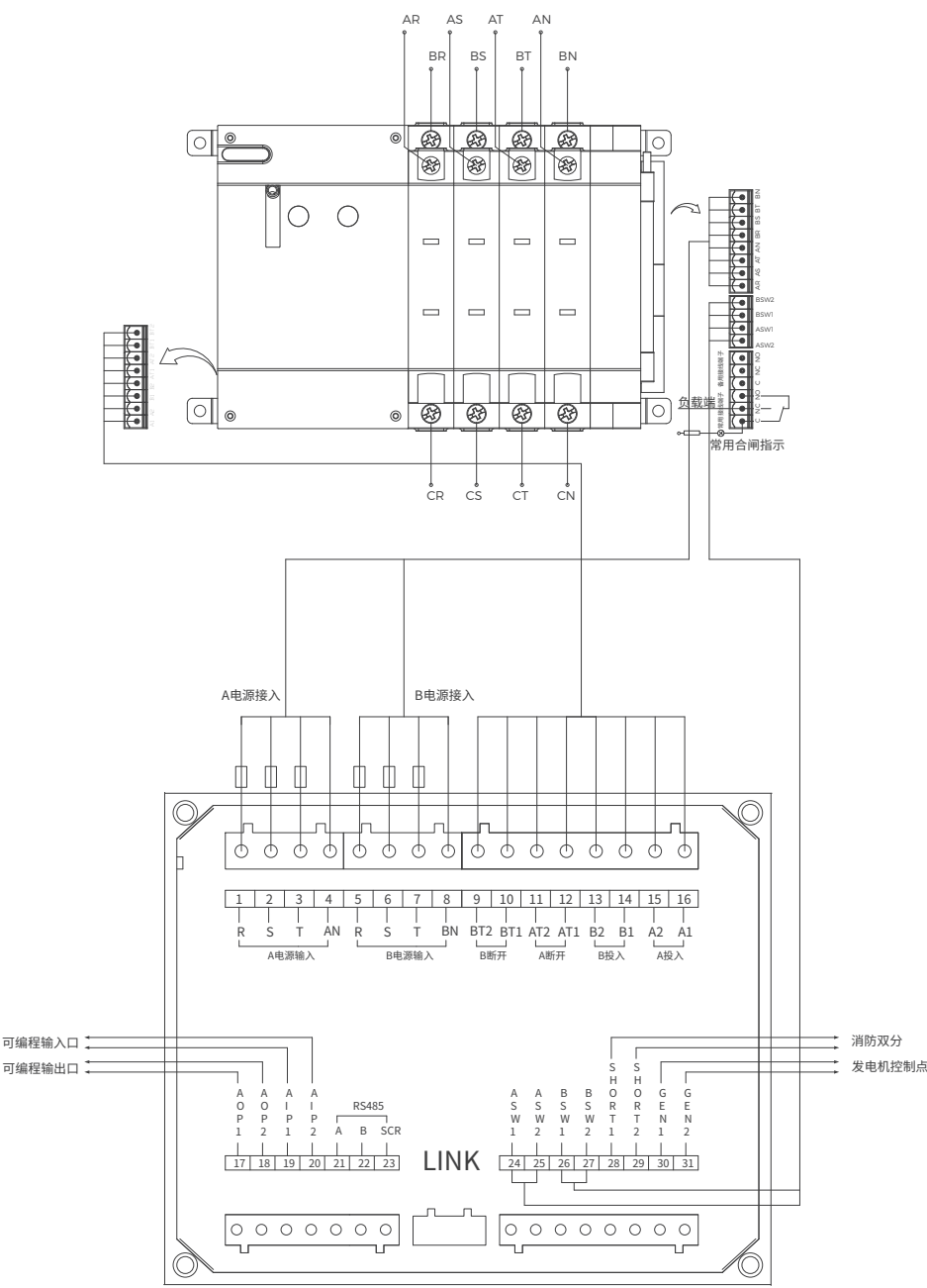
BQ3-63-III 16A~63A H 型控制器与三段式切换开关的接线图
