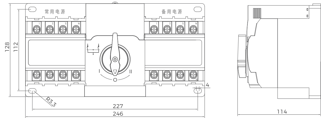
BQ1A-63/125G 外形、安装尺寸及接线图（基本型、J 型和 D 型外观大小及接线方式一致）
