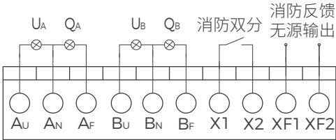
外接端子接线图
