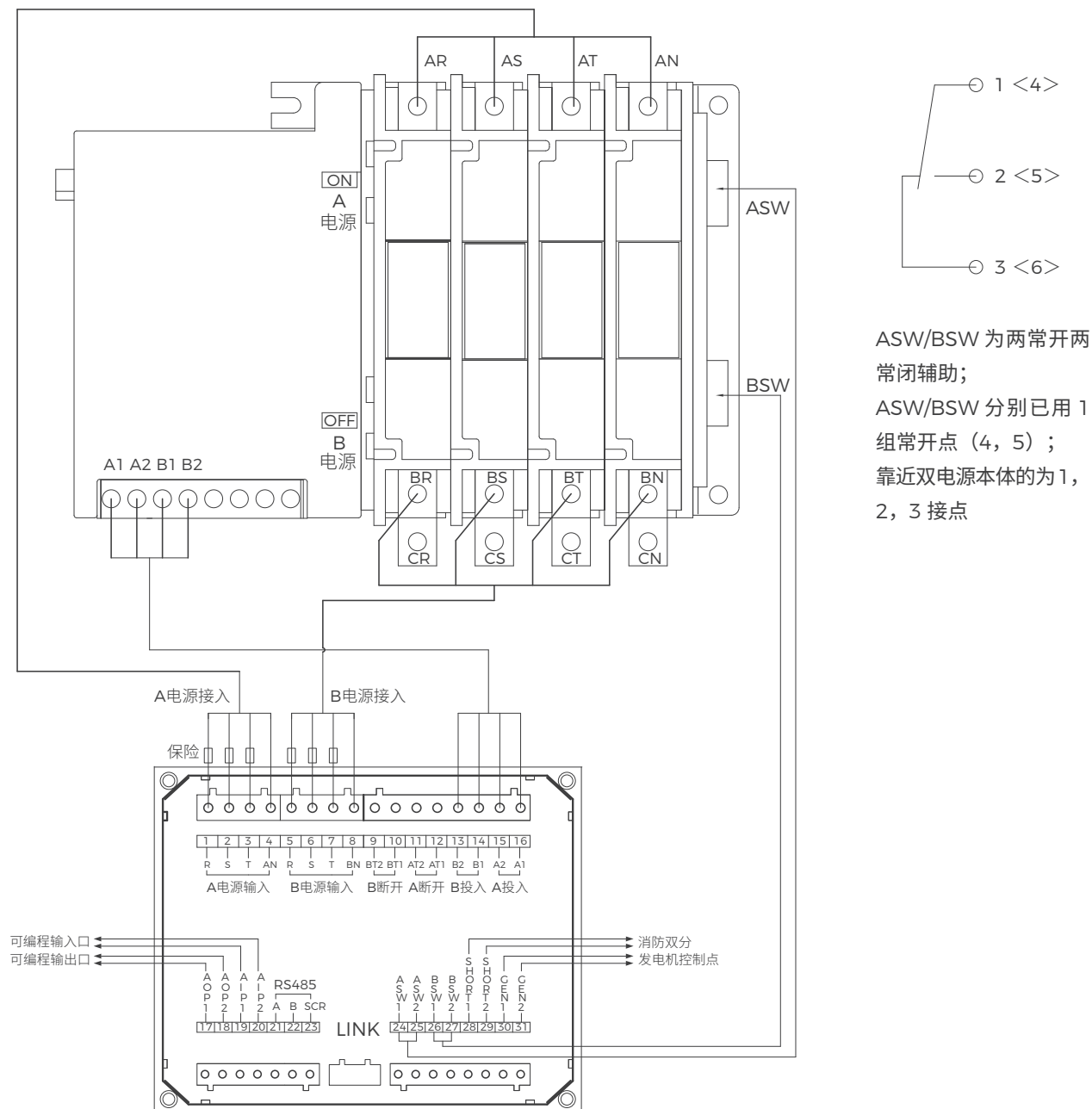
BQ3-63-II 80A~5000A H 型控制器与二段式切换开关的接线图
