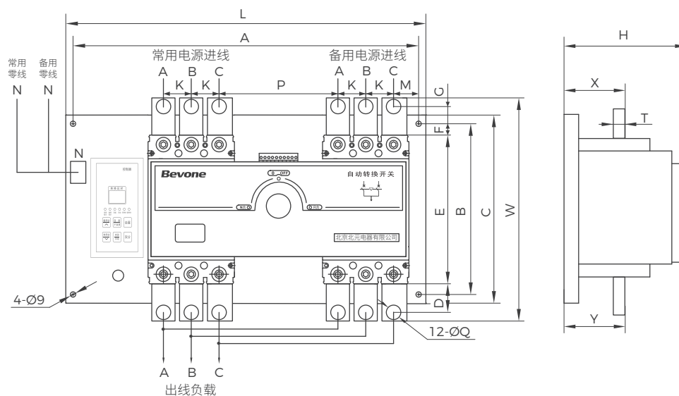
BM30Q1-400~800/3P 外形、安装尺寸及接线图
