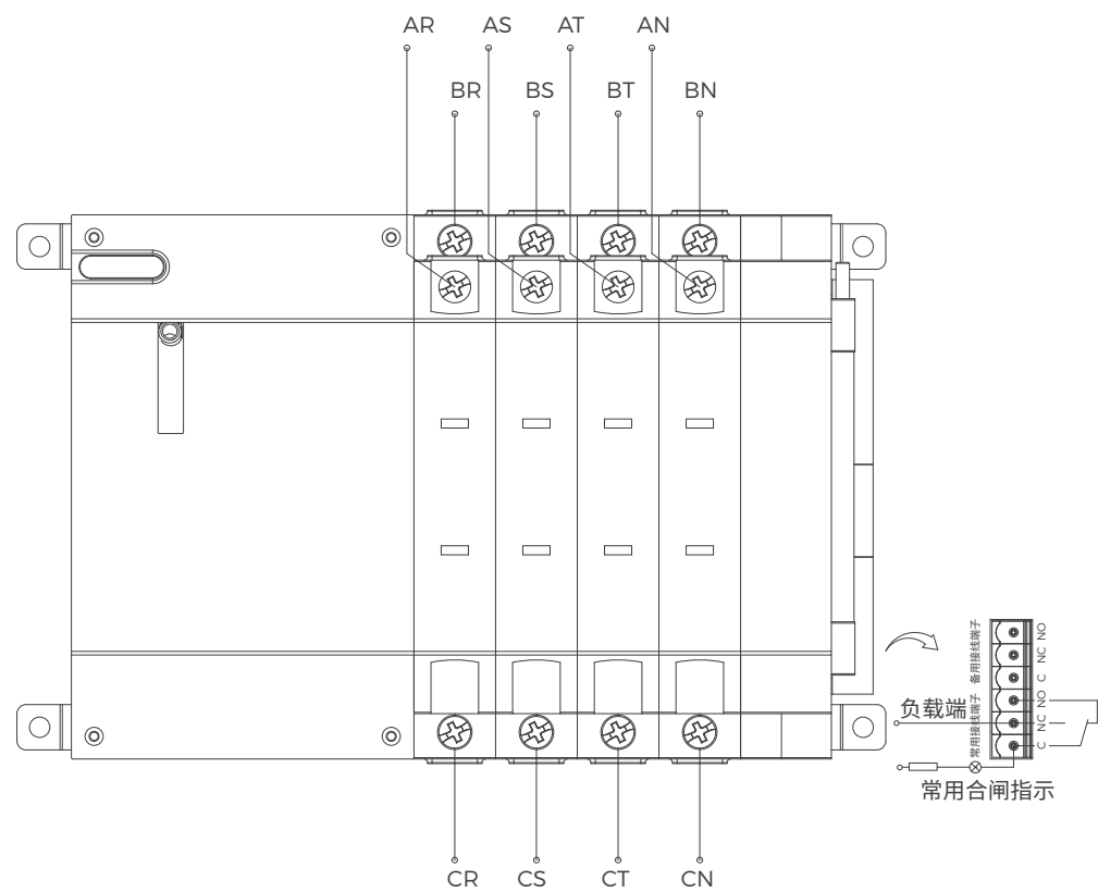
BQ3-16A~63A N 型控制器接线图
