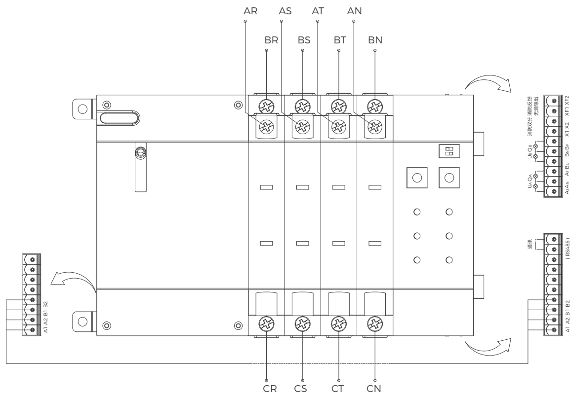
BQ3-63-II 16A~63A J 型控制器与二段式切换开关的接线图
