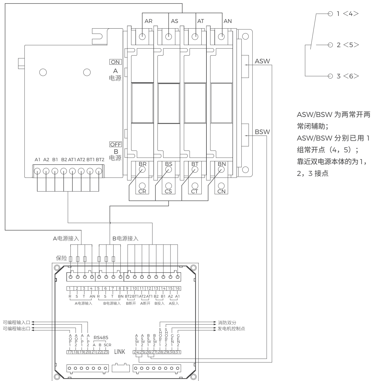
BQ3-63-III 80A~5000A H 型控制器与三段式切换开关的接线图
