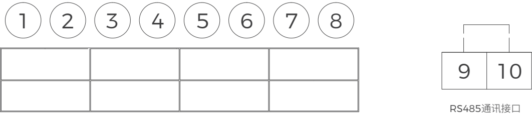
9.1 基本型外接端子图
