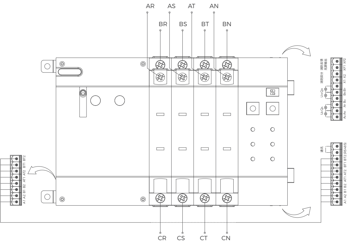
BQ3-III 16A~63A J 型控制器与三段式切换开关的接线图
