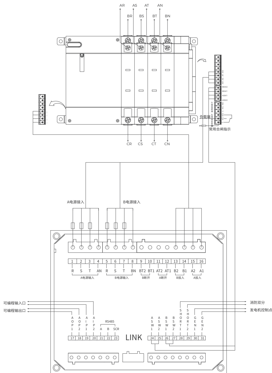
BQ3-63-II 16A~63A H 型控制器与二段式切换开关的接线图
