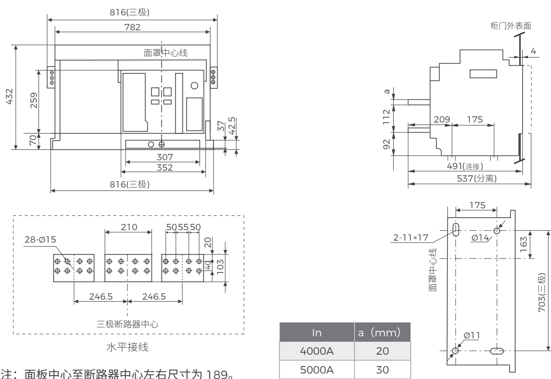
图 48 抽屉式断路器安装尺寸及外形尺寸 (BW1A-6300 4000/3P、BW1A-6300 5000/3P)
