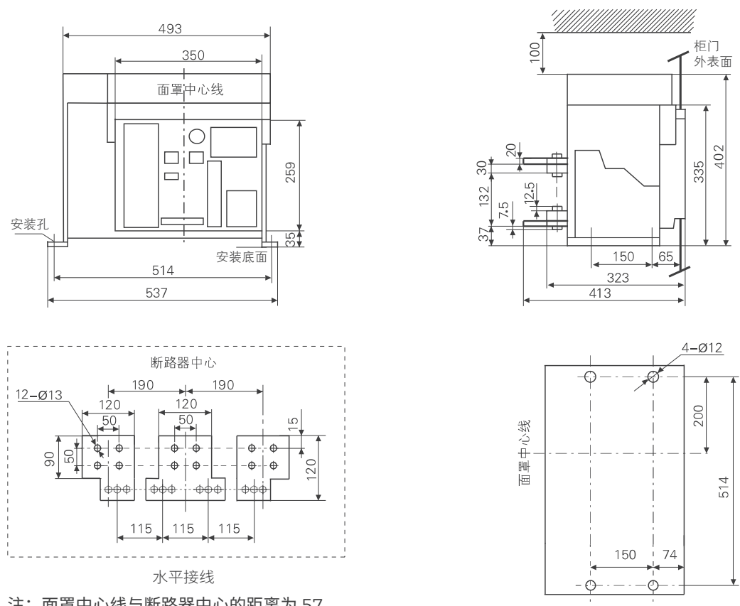
图 40 固定式断路器安装尺寸及外形尺寸 (BW1A-4000/3)
