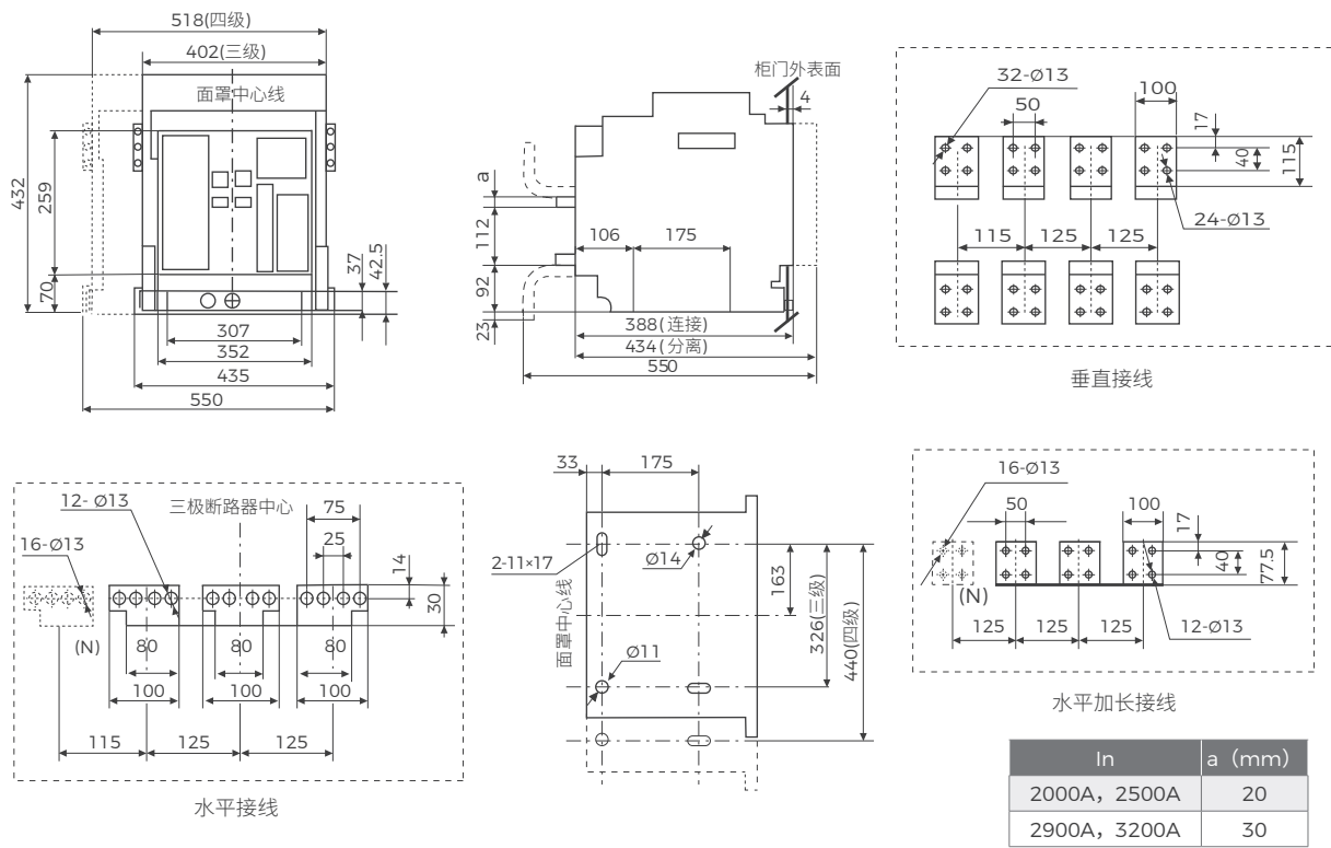
图 45 抽屉式断路器安装尺寸及外形尺寸 (BW1A-3200)
