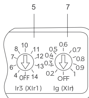
BM30E-630, I_n=630A 电子式脱扣器 (C 型接地保护)
