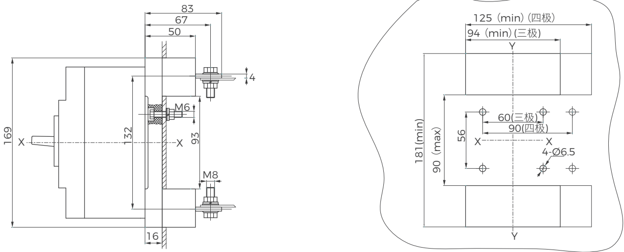
BM30E-100M/H 塑壳断路器插入式板后接线
