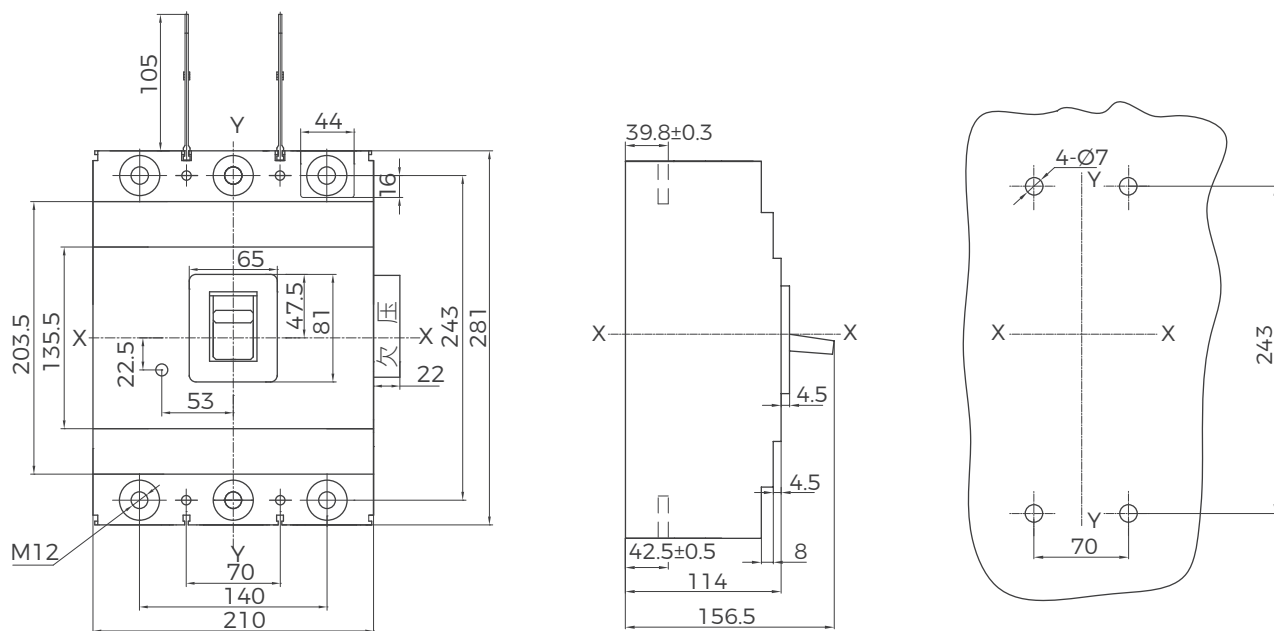
BM30-630H、BM30-800 (M、H) 板前接线 (三极)
