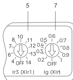
BM30E-800, I_n=630A 电子式脱扣器 (C 型接地保护)
