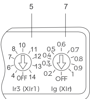
BM30E-800, I_n=800A 电子式脱扣器 (C 型接地保护)
