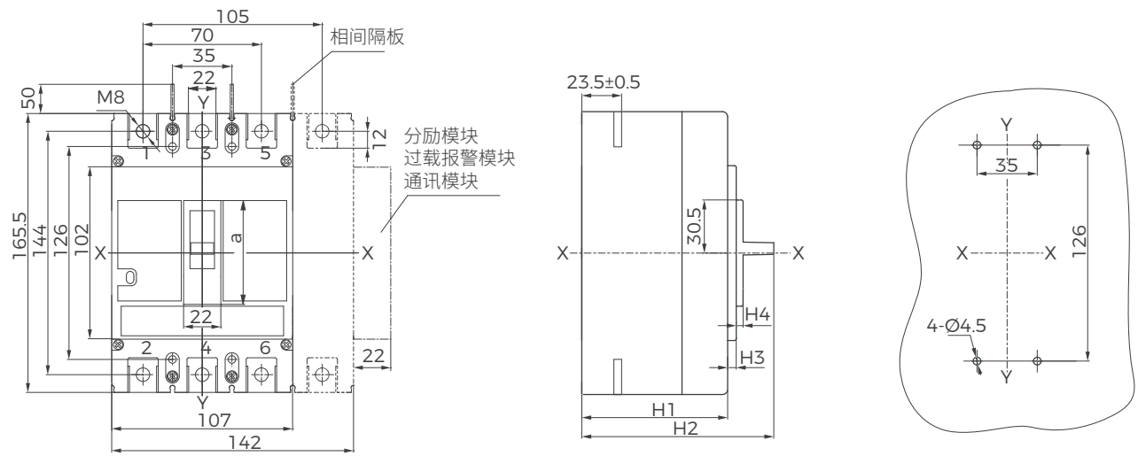
BM30E-250M/H 塑壳断路器板前接线
