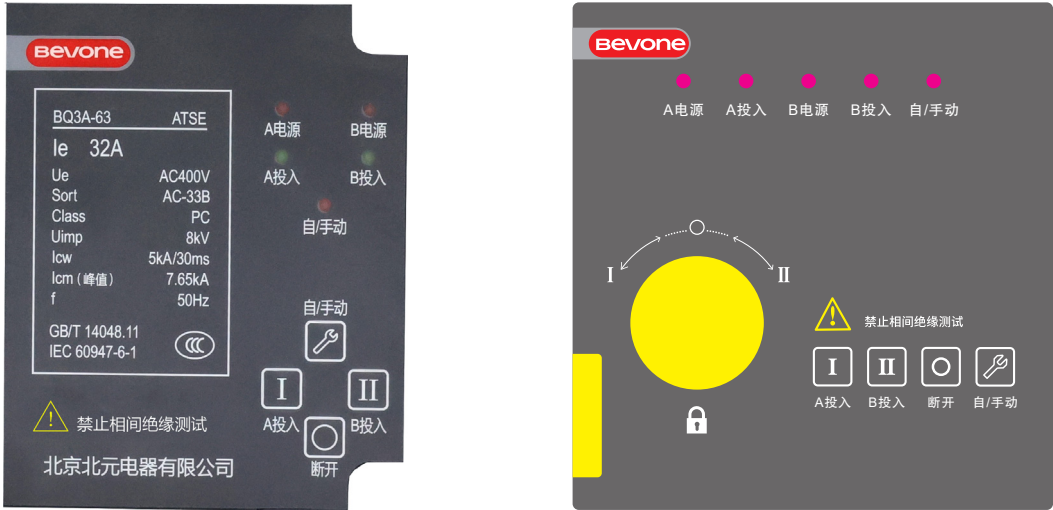
图 1 J 型控制器面板示意图（左图为 63 壳架，右图为 125-800 壳架）
