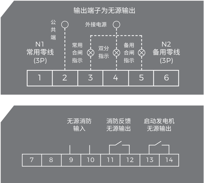
图 8 J 型产品外接端子接线图
