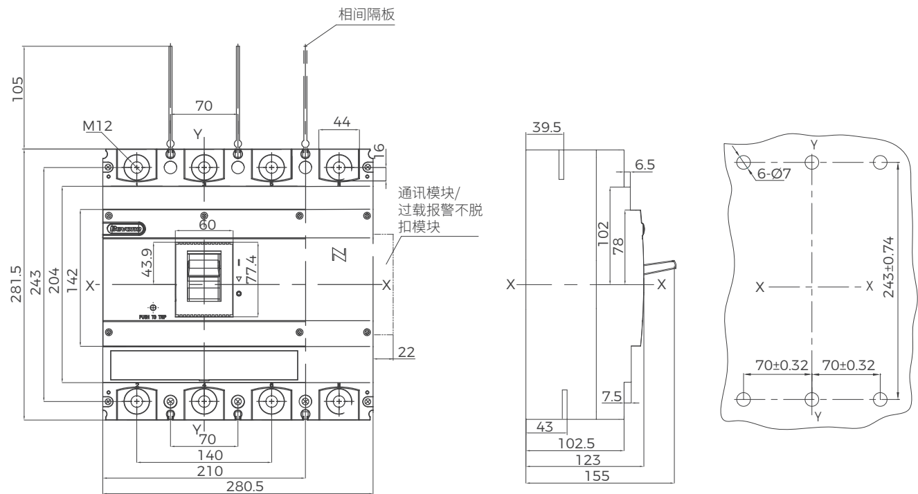
BM3E-630L/M/H 塑壳断路器板前接线
