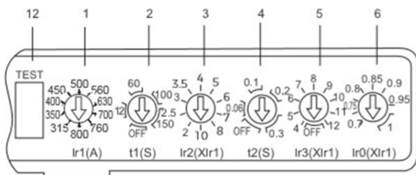
BM3E-800, In=800A 电子式脱扣器
