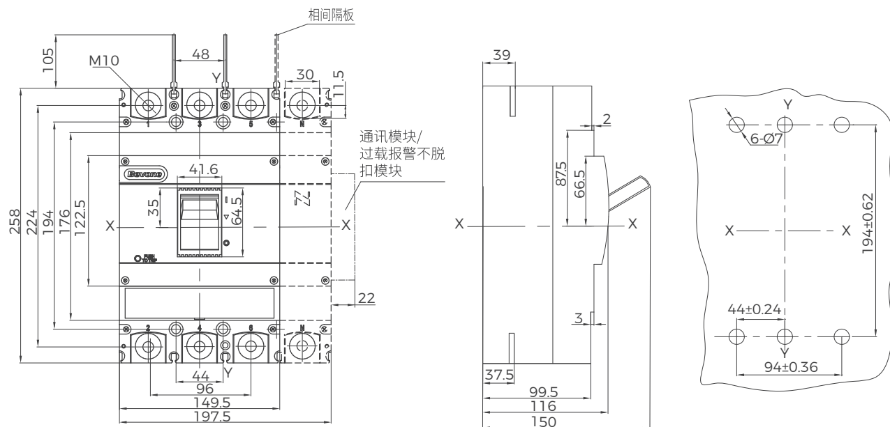
BM3E-400C/L/M/H 塑壳断路器板前接线
