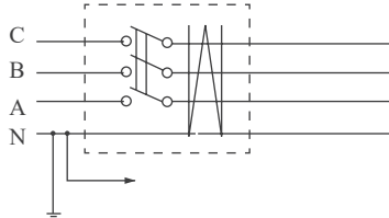
正确接线
