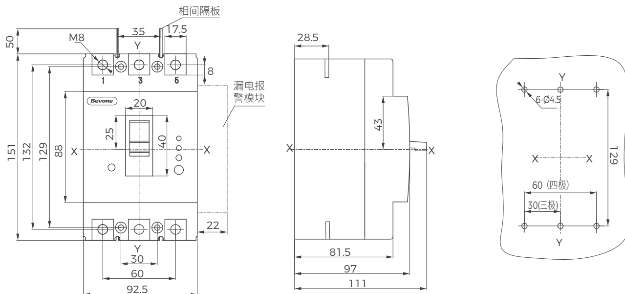
BM3L-125 (三极)
