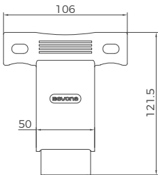
加长手柄外形尺寸图
