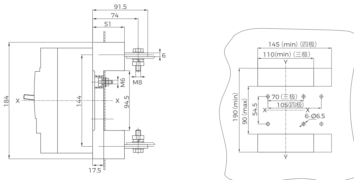
BM3E-250C/L/M/H 塑壳断路器插入式板后接线
