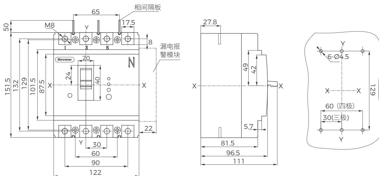
BM3L-125 (四极)
