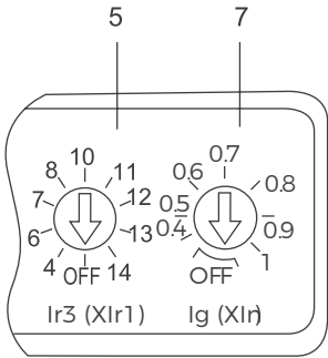
BM3E-125, In=32A 电子式脱扣器 (C 型接地保护)
