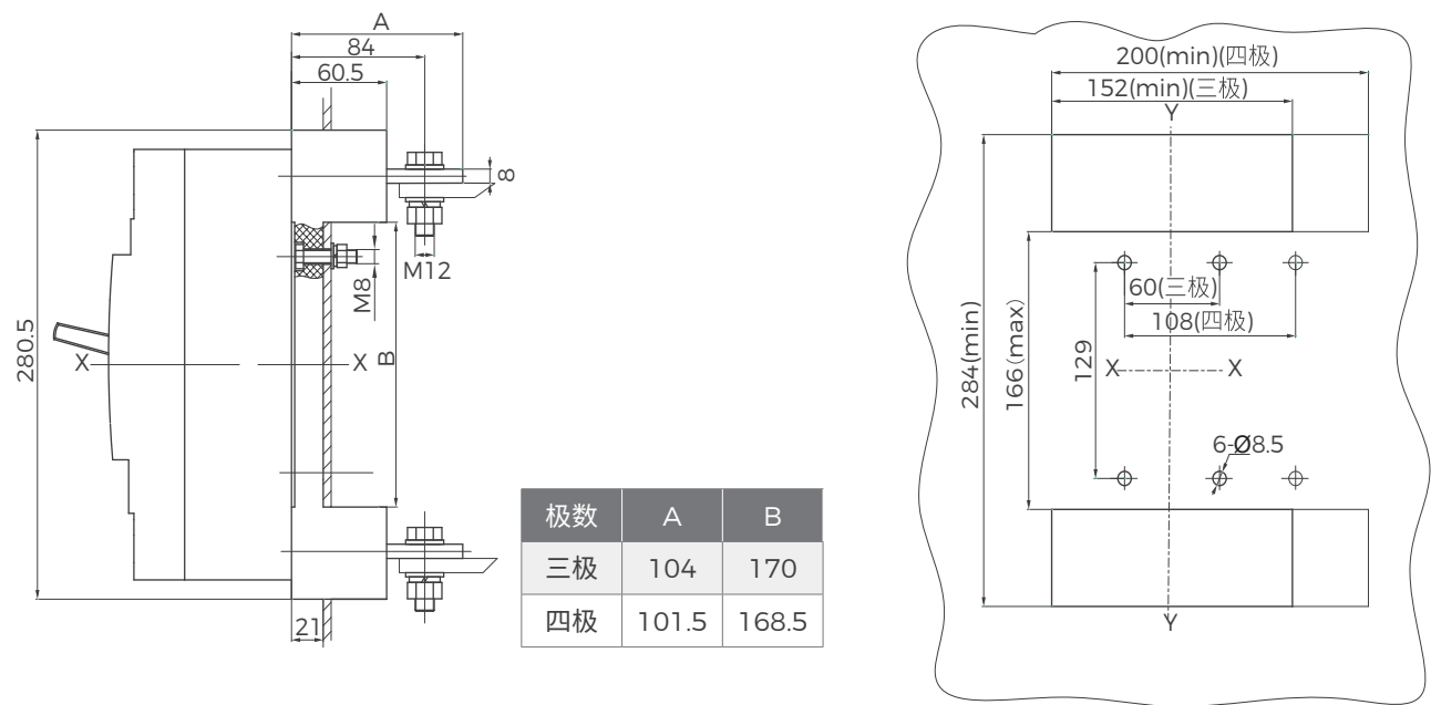
BM3E-630L/M/H 塑壳断路器板前接线
