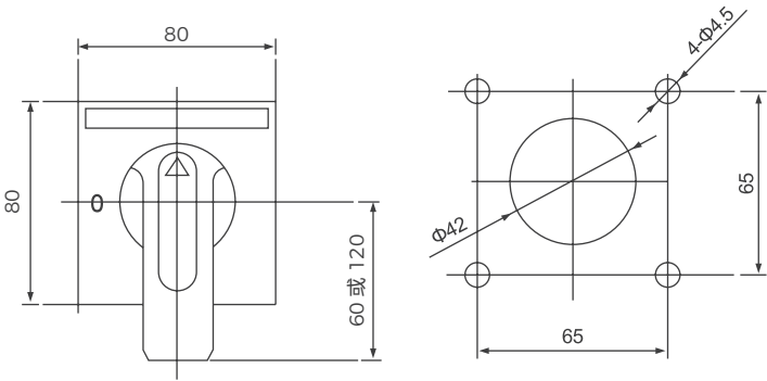
“F”型方形手柄外形及门板开孔尺寸 (开孔中心离铰链距离不小于 200mm)
