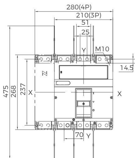
BM3E-1600 塑壳断路器板前接线
