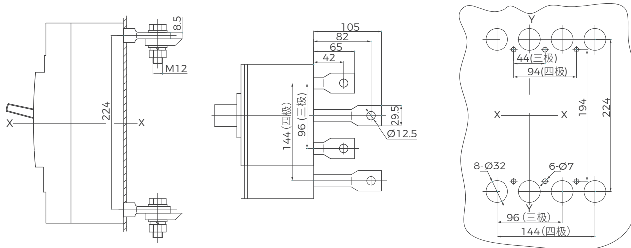
BM3E-400C/L/M/H 塑壳断路器板后接线
