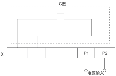
外挂欠电压脱扣器模块接线图
