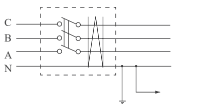
错误接线
