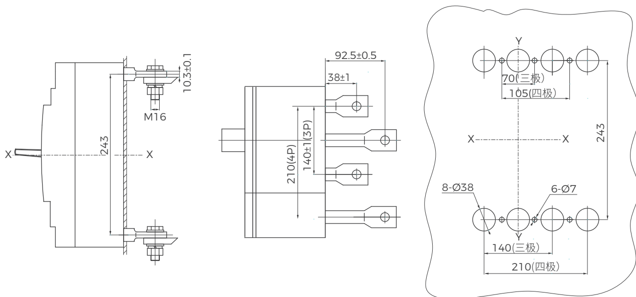
BM3E-630L/M/H 塑壳断路器板后接线
