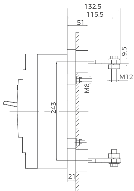
BM3E-800L/M/H 4P 塑壳断路器插入式板后接线
