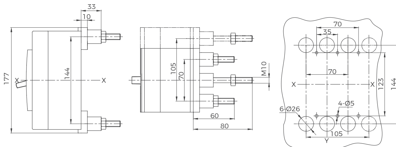
BM3E-250C/L/M/H 塑壳断路器板后接线
