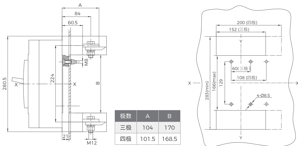
BM3-400 (C、L、M、H) 插入式板后接线 (三极、四极)
