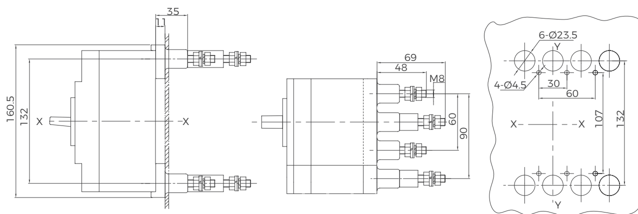
BM3E-125C/L/M/H 塑壳断路器板后接线
