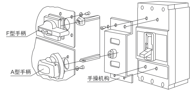
手操机构安装示意图
