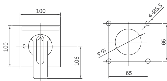
1250 壳架“F”型方形手柄外形及门板开孔尺寸 (开孔中心离铰链距离不小于 100mm)
