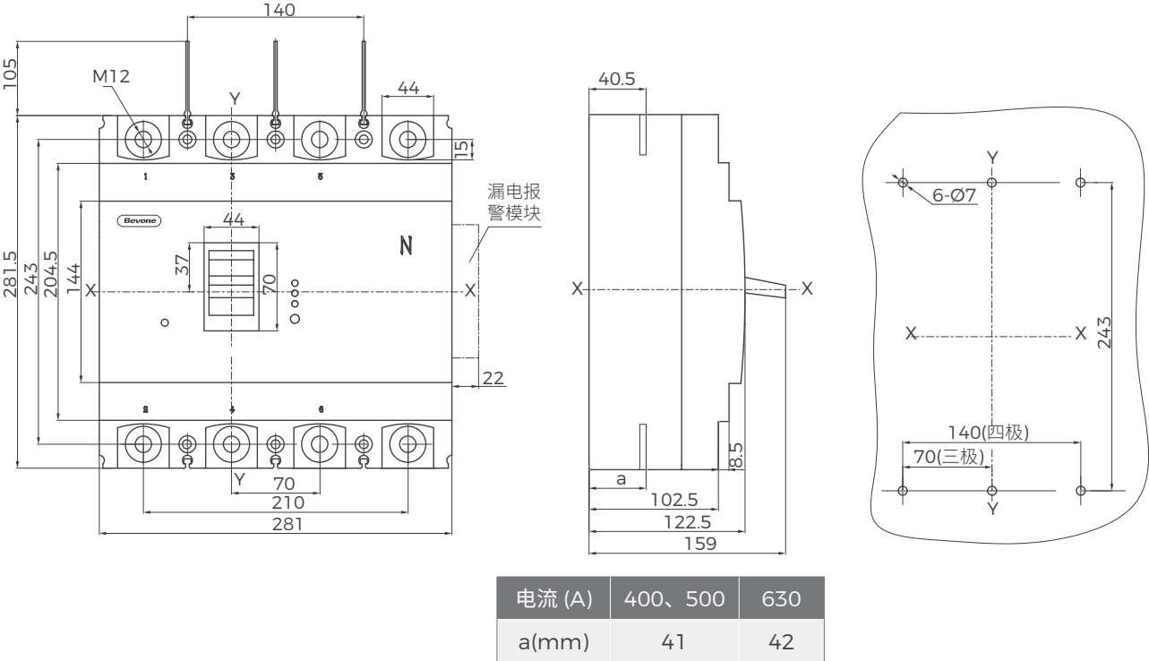
BM3L-630（四极）
