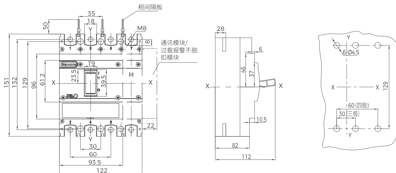
BM3E-125C/L/M/H 塑壳断路器板前接线
