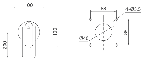
1600 壳架“F”型手柄外形及门板开孔尺寸
