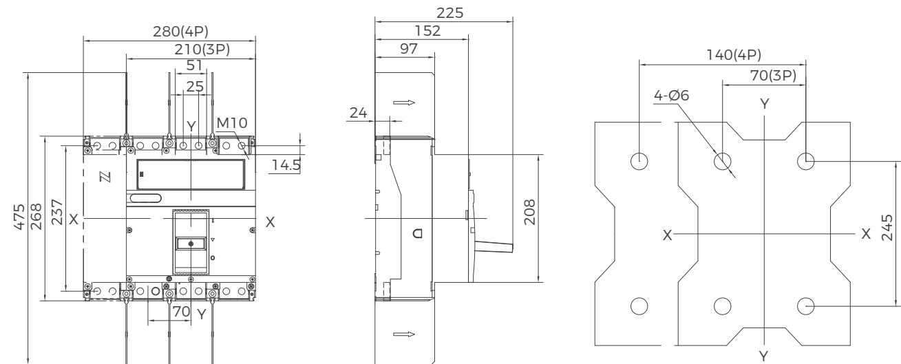
BM3-1600( 三极、四极 )
