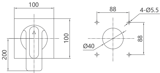
1600 壳架“F”型手柄外形及门板开孔尺寸
