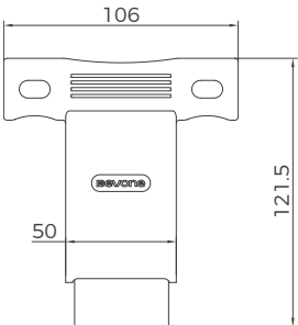
加长手柄外形尺寸图
