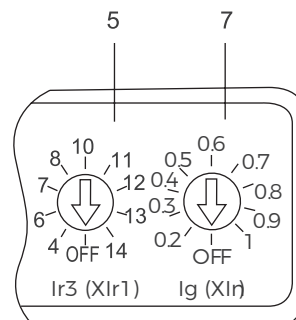
BM3E-630, In=630A 电子式脱扣器 (C 型接地保护)
