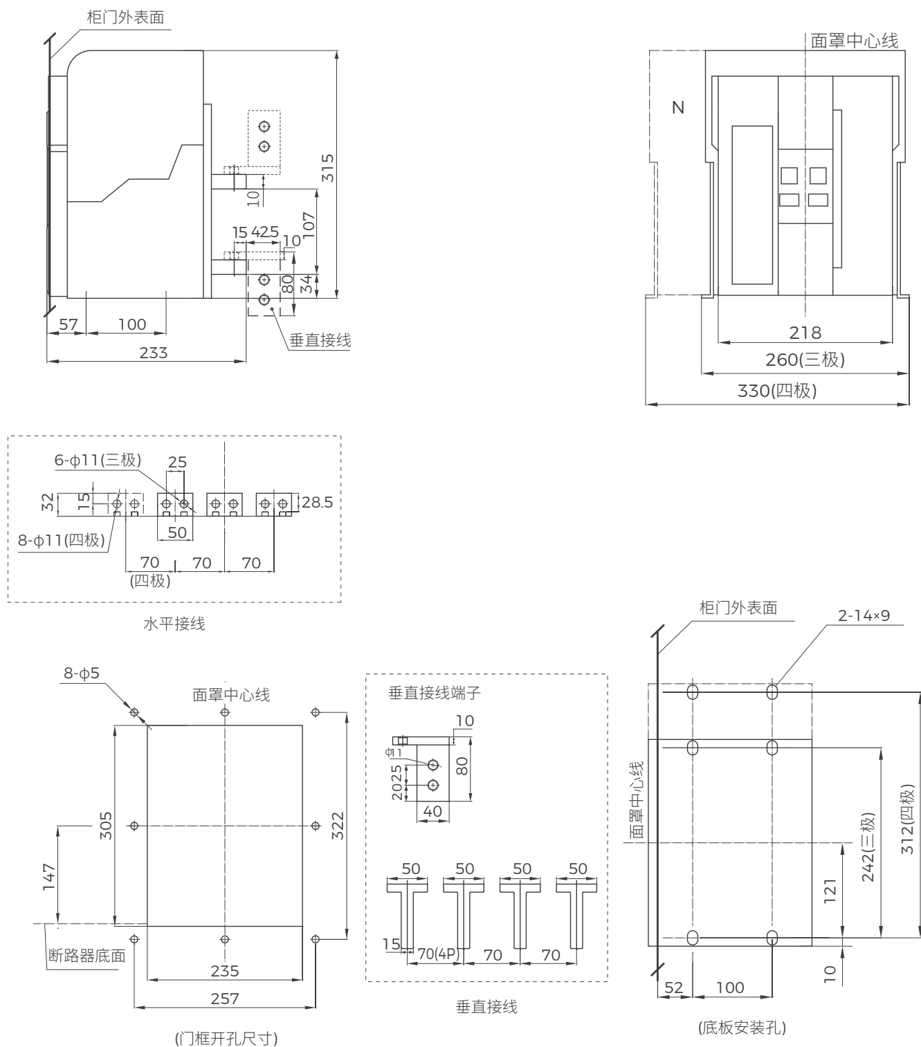
图 37 固定式断路器安装尺寸及外形尺寸 (BW1-1600)
