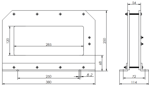
图 26-1 BH-LMB-280×120 互感器
