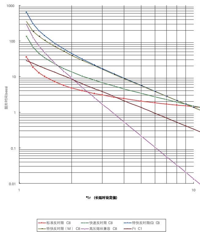
不同曲线类型对比（曲线速率：C8）
