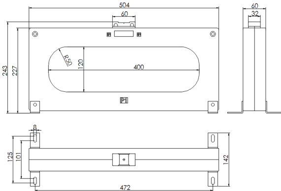
图 26-2 ZCT1-400 互感器
