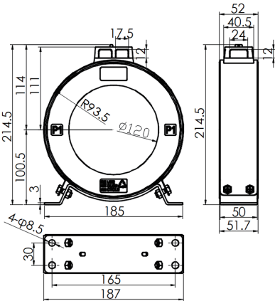
图 25-2 ZT120 互感器
