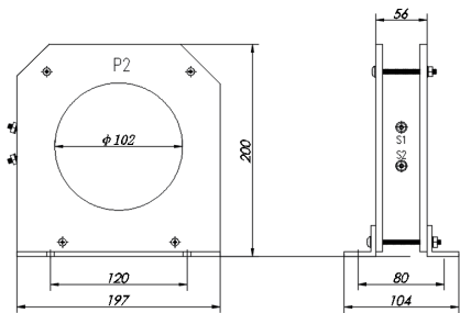
图 25-1 100LDJ1 互感器
