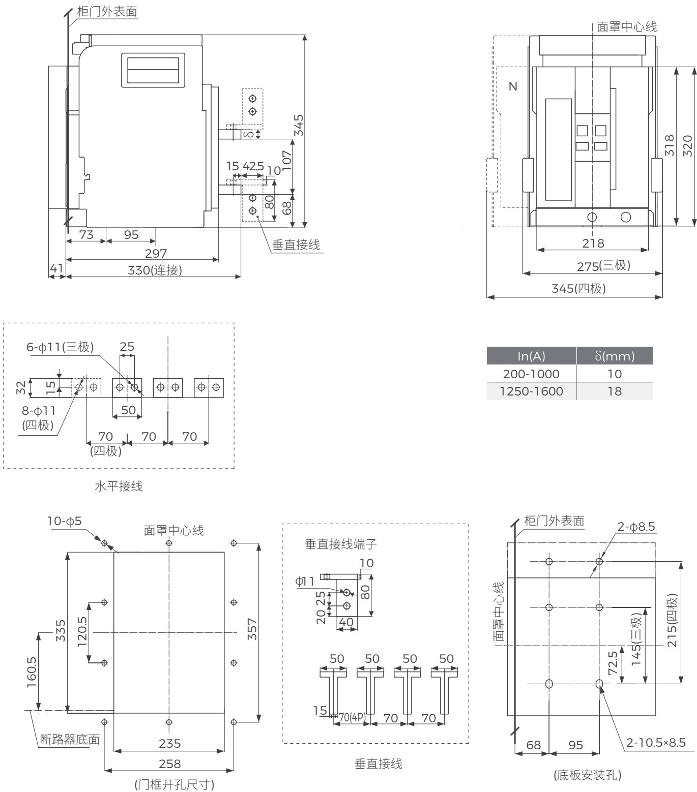
图 43 抽屉式断路器安装尺寸及外形尺寸 (BW1-1600)
