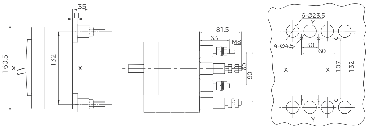
BM3-125 (C、F、L、N、M、S、H) /BM3-160 (C、L、N、M、S) 板后接线 (三极、四极)
