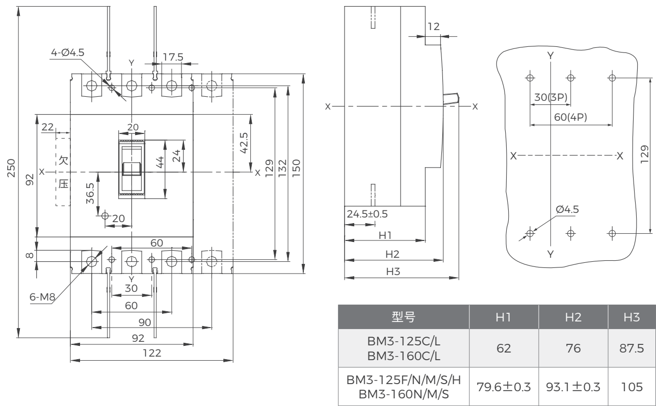
BM3-125 (C、F、L、N、M、S、H) /BM3-160 (C、L、N、M、S) 板后接线 (三极、四极)
