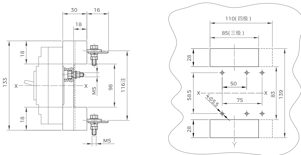
BM3-63(L、M) / BM3-100C 插入式板后接线 (三极、四极)
