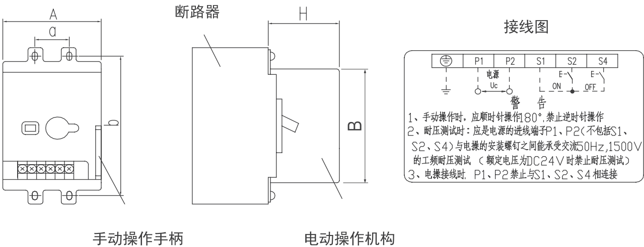
外形尺寸和技术参数
