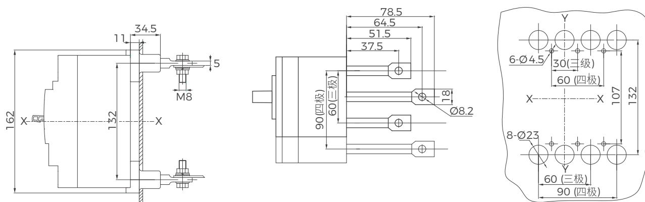
BM3E-125C/L/M/H 塑壳断路器板后接线
