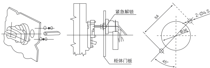
“A”型圆形手柄外形及门板开孔尺寸 (开孔中心离铰链距离不小于 200mm)
