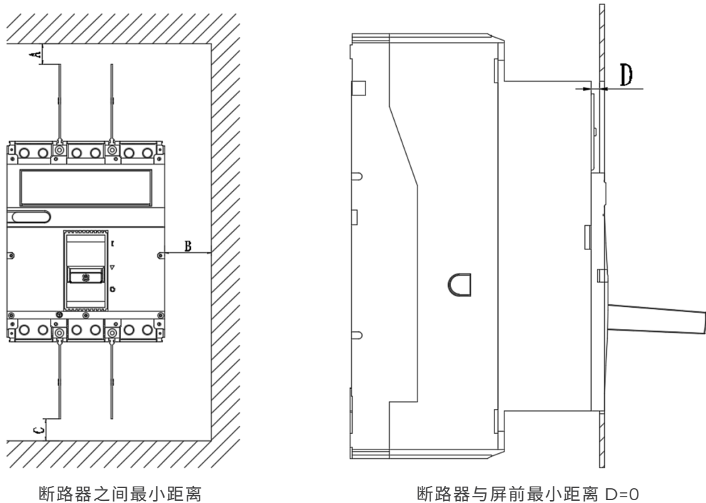
断路器安全距离
