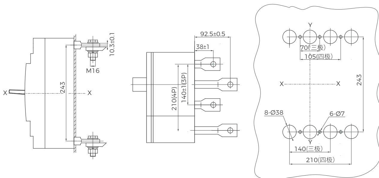
BM3E-800L/M/H 塑壳断路器板后接线
