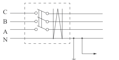
错误接线
