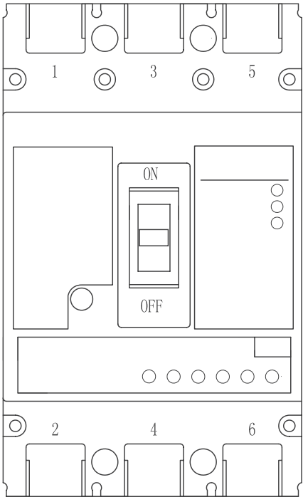
BM30E-100, In=32A 电子式脱扣器
