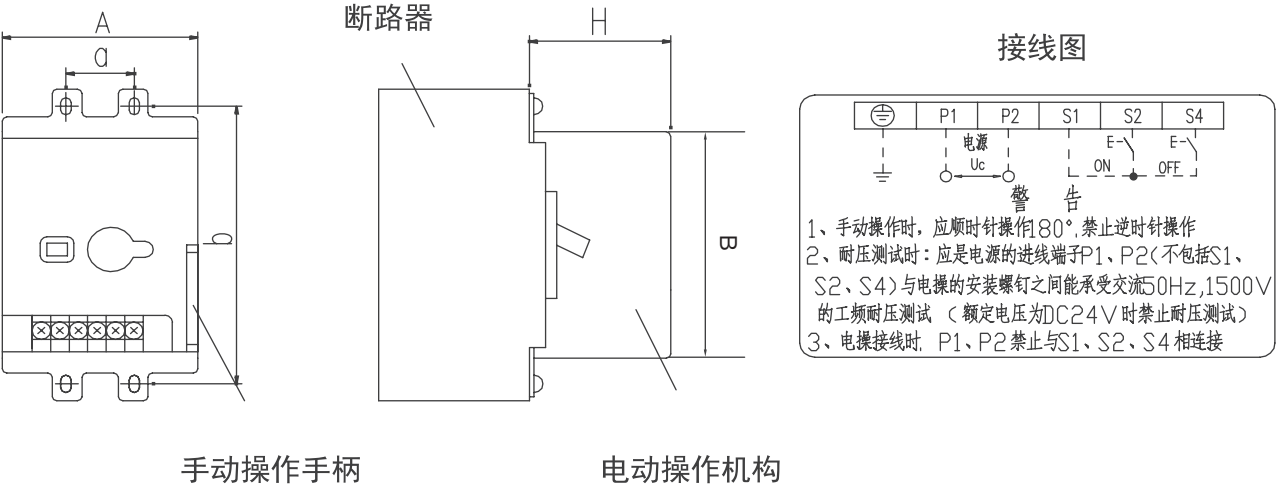
外形和安装示意图
