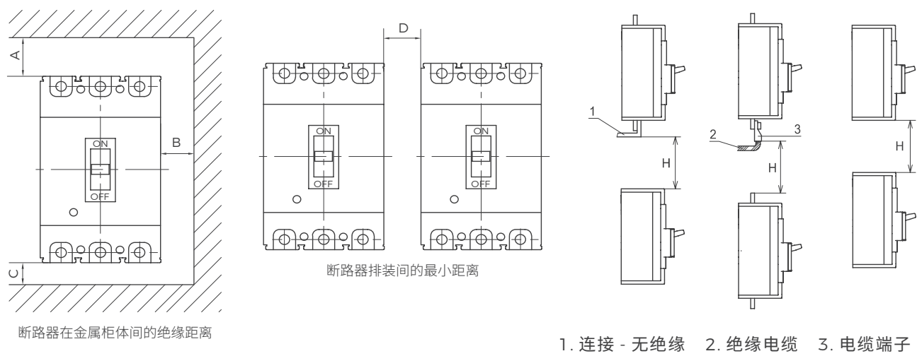
BM30 系列塑料外壳式断路器安全距离 (mm)
