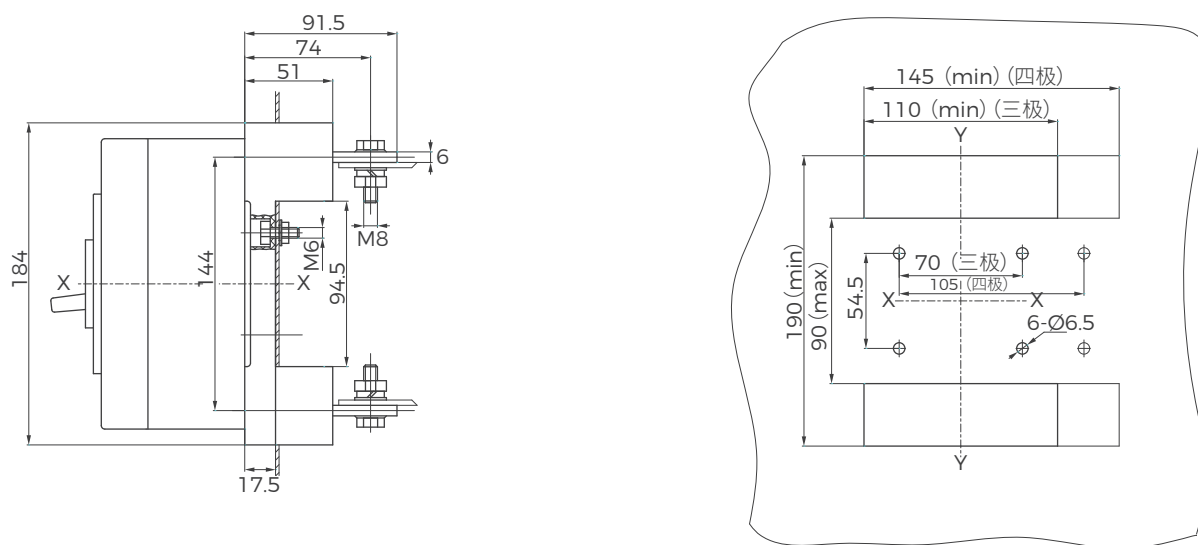
BM30E-250M/H 塑壳断路器插入式板后接线
