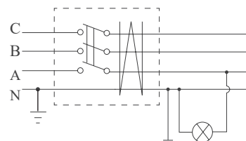
错误接线
