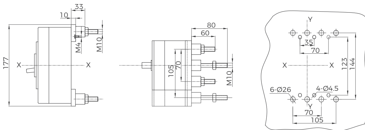
BM30E-250M/H 塑壳断路器板后接线
