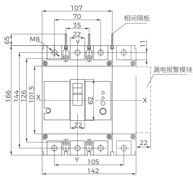
BM30L-250（三极、四极）
