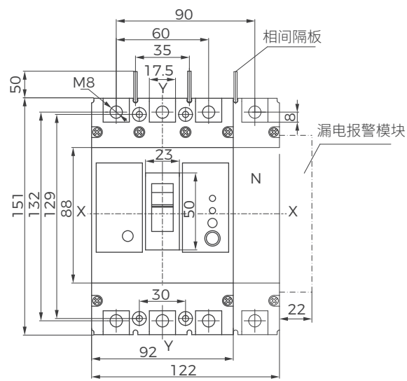
BM30L-125（三极、四极）
