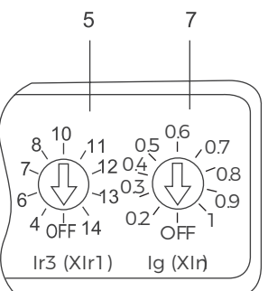
BM30E-250, In=250A 电子式脱扣器 (G 型接地保护)
