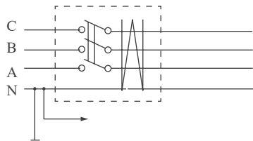
正确接线
