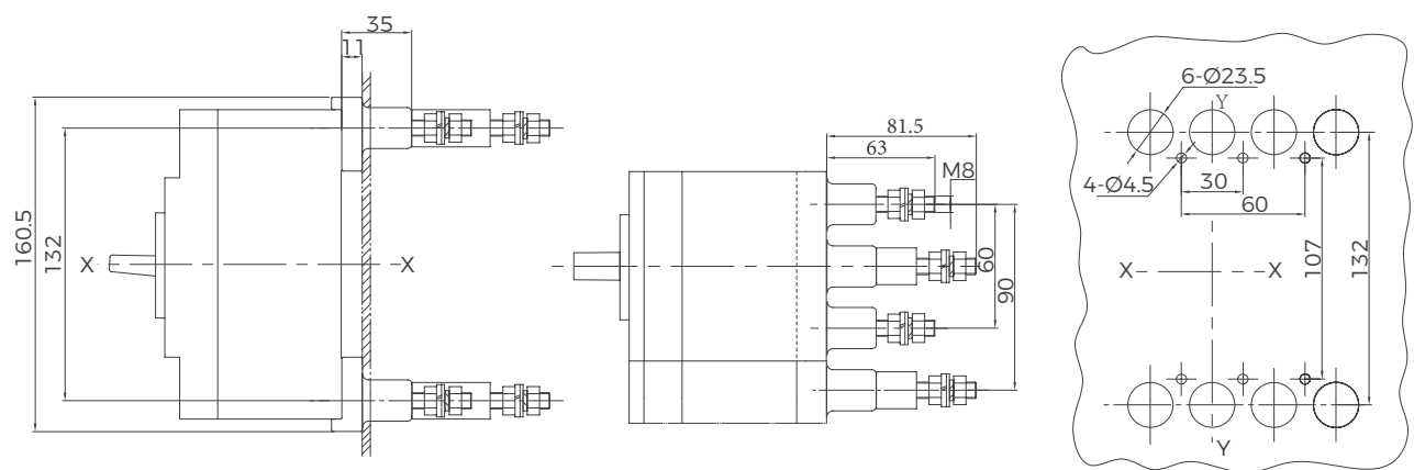
BM30E-100M/H 塑壳断路器板后接线
