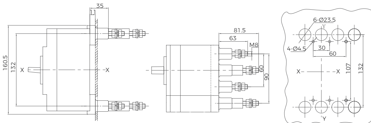
BM30-125 (L、M、H)、BM30-160 (L、M) 板后接线 (三极、四极)
