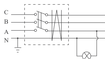
正确接线
