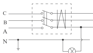
错误接线
