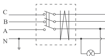
正确接线
