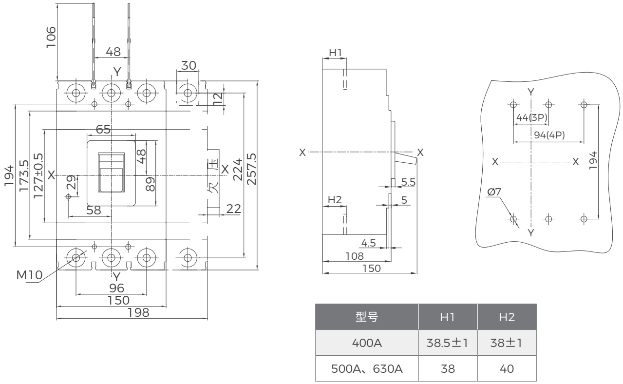
BM30-400 (L、M、H) BM30-630 (L、M) 板前接线 (三极、四极)
