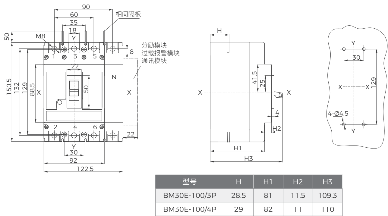
BM30E-100M/H 塑壳断路器板前接线
