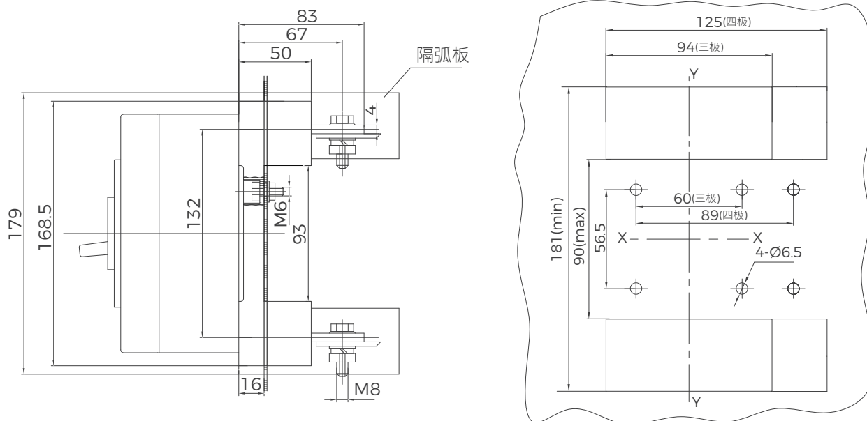
BM30-125 (L、M、H)、BM30-160 (L、M) (10-125A) 插入式板后接线 (三极、四极)
