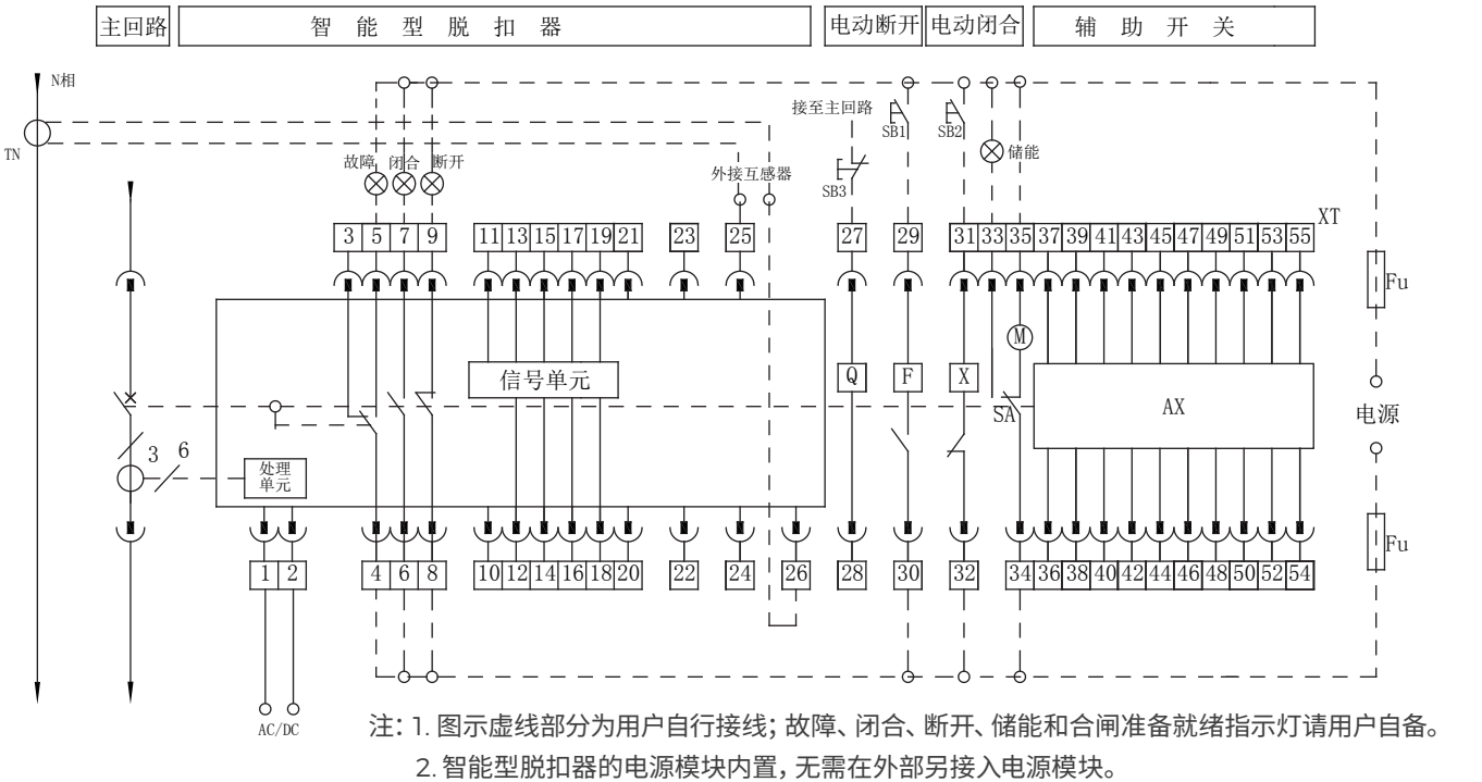
4 开 4 闭转换 (T4)
