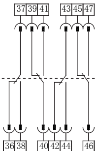
5 开 5 闭转换 (T5)
