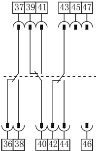
4 开 4 闭转换 (T4)
