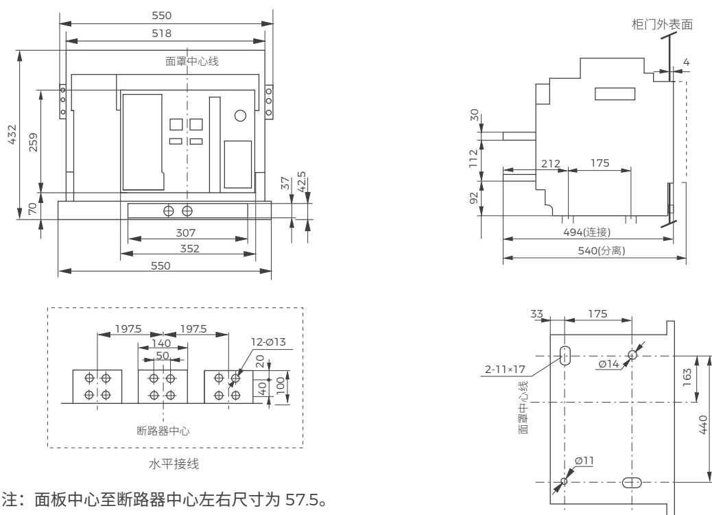
图 46 抽屉式断路器安装尺寸及外形尺寸 (BW1A-4000/3)
