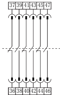
4 开 4 闭独立 (D4)
