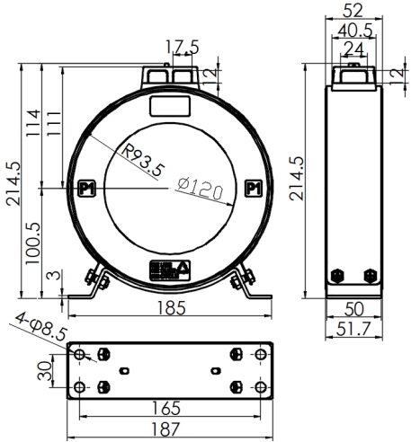
图 25-2 ZT120 互感器
