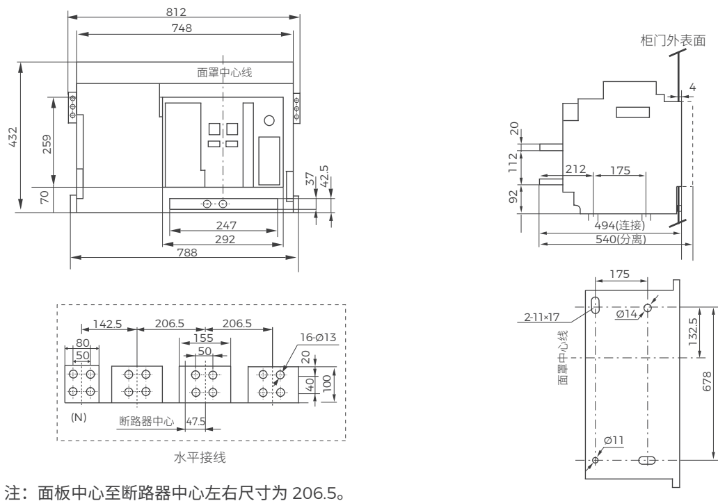
图 47 抽屉式断路器安装尺寸及外形尺寸 (BW1A-4000/4)
