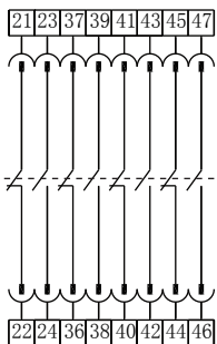
5 开 5 闭独立 (D5)
