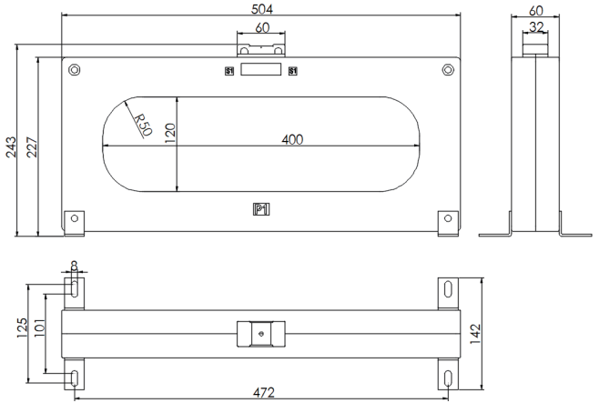
图 26-2 ZCT1-400 互感器
