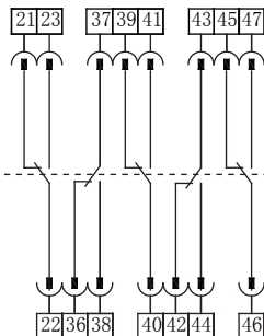
6 开 6 闭转换 (T6)
