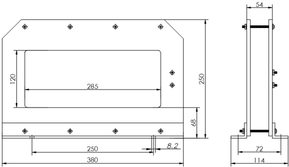
图 26-1 BH-LMB-280×120 互感器
