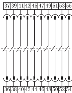
6 开 6 闭独立 (D6)
