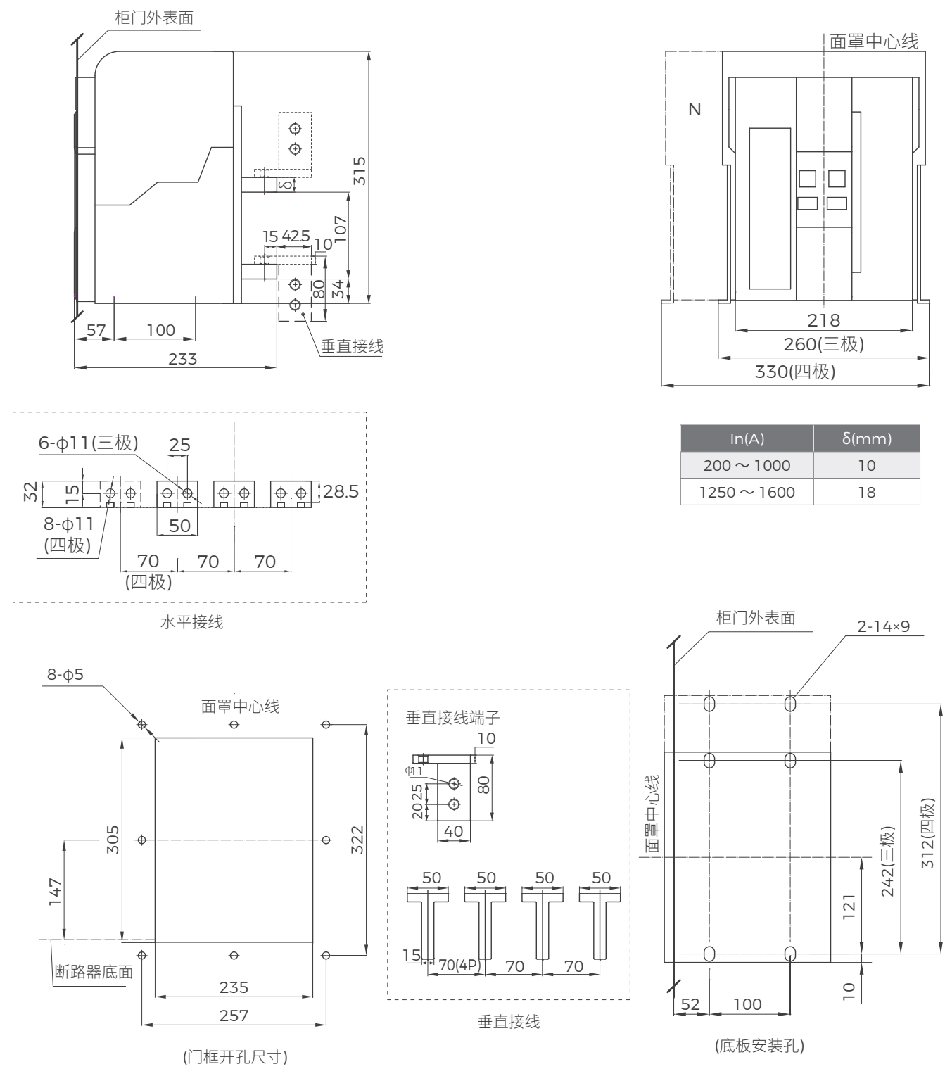
BW1A-1600 固定式断路器外形及安装尺寸
