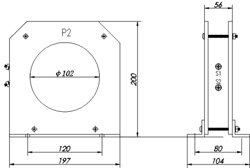
图 25-1 100LDJ1 互感器
