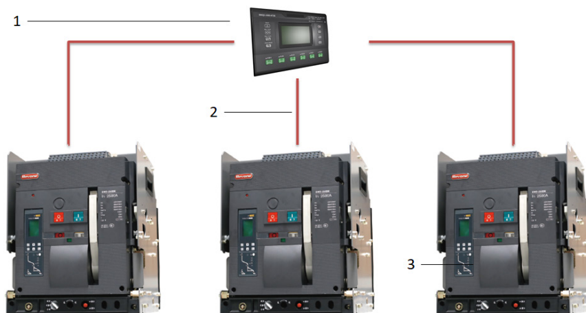
1、控制器 2、电气联锁线束 3、执行断路器
