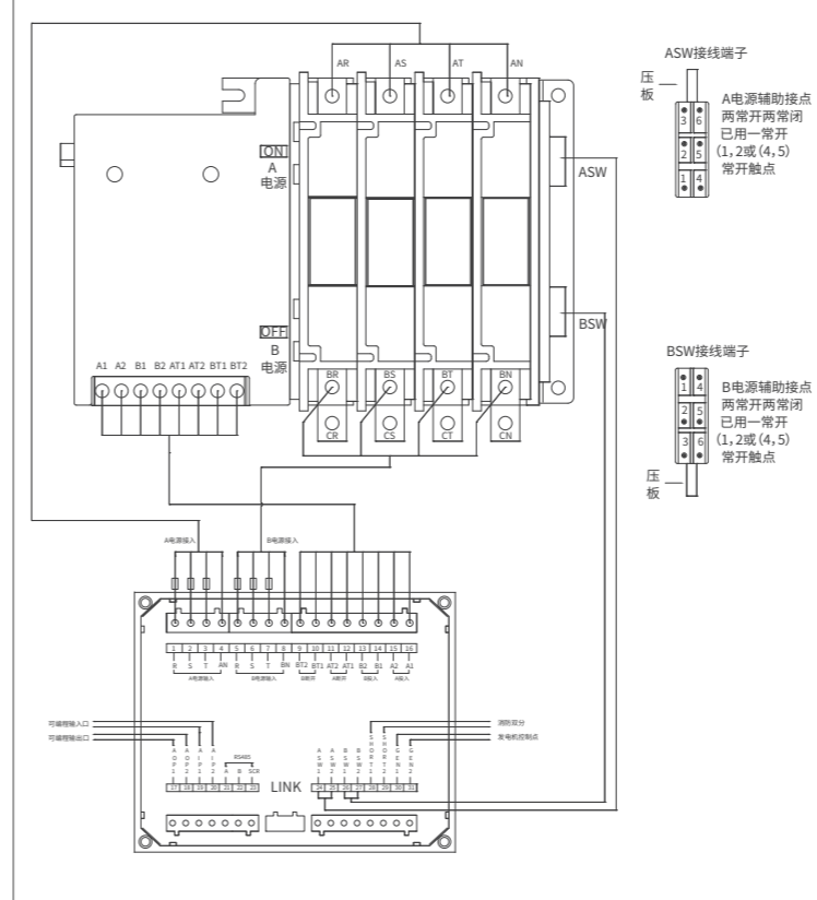
H型控制器与三段式切换开关的接线图
