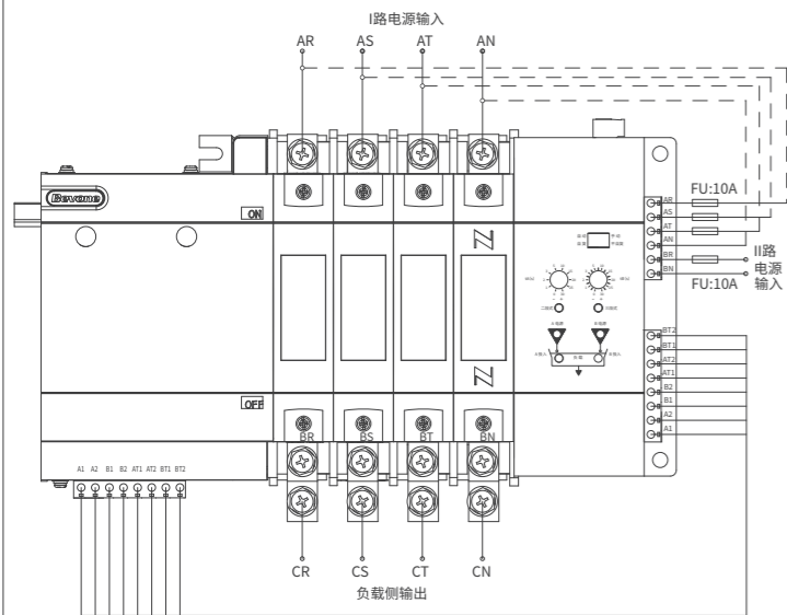
J型控制器与三段式切换开关的接线图
