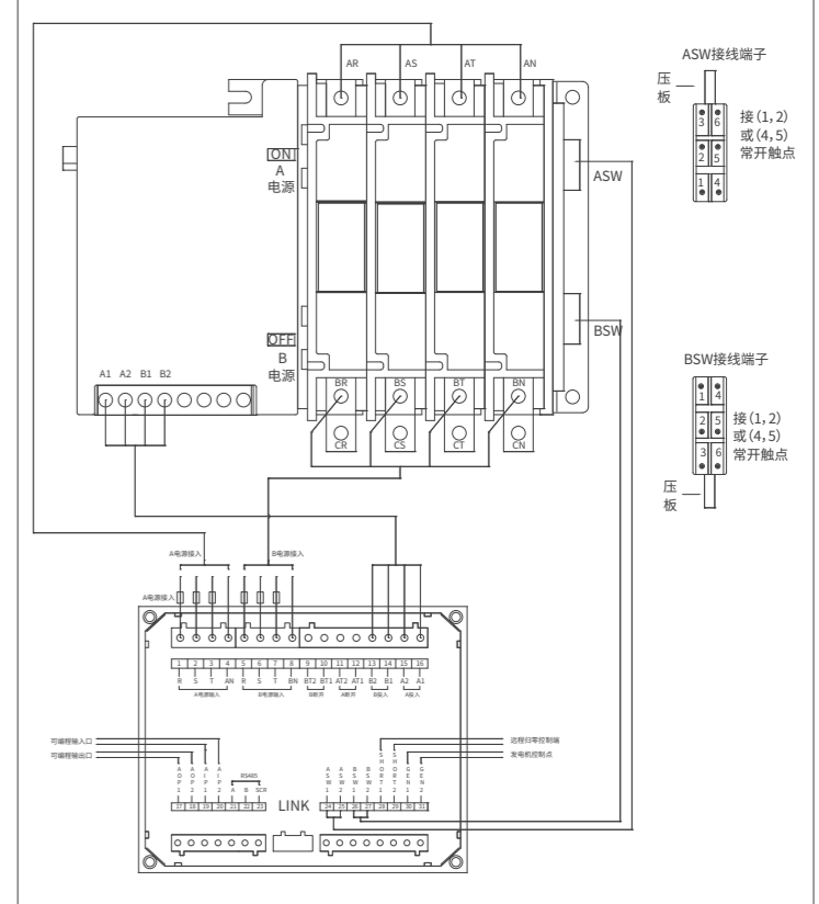
H型控制器与二段式切换开关的接线图
