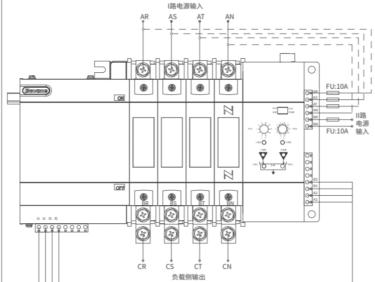
J型控制器与二段式切换开关的接线图
