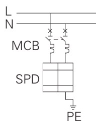
2P 产品接线图
