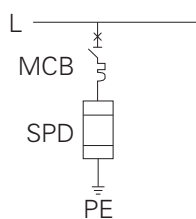
1P 产品接线图
