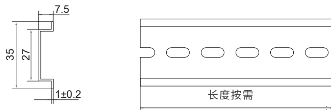
安装导轨尺寸
