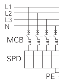
4P 产品接线图
