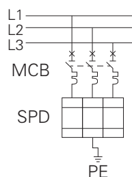
3P 产品接线图
