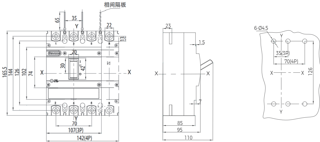
BM3E-250M/H 塑壳断路器板前接线
