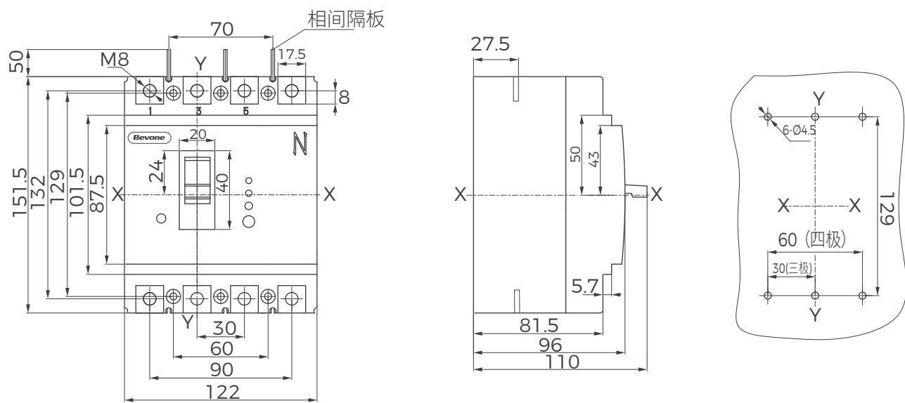
BM3L-125 (四极)
