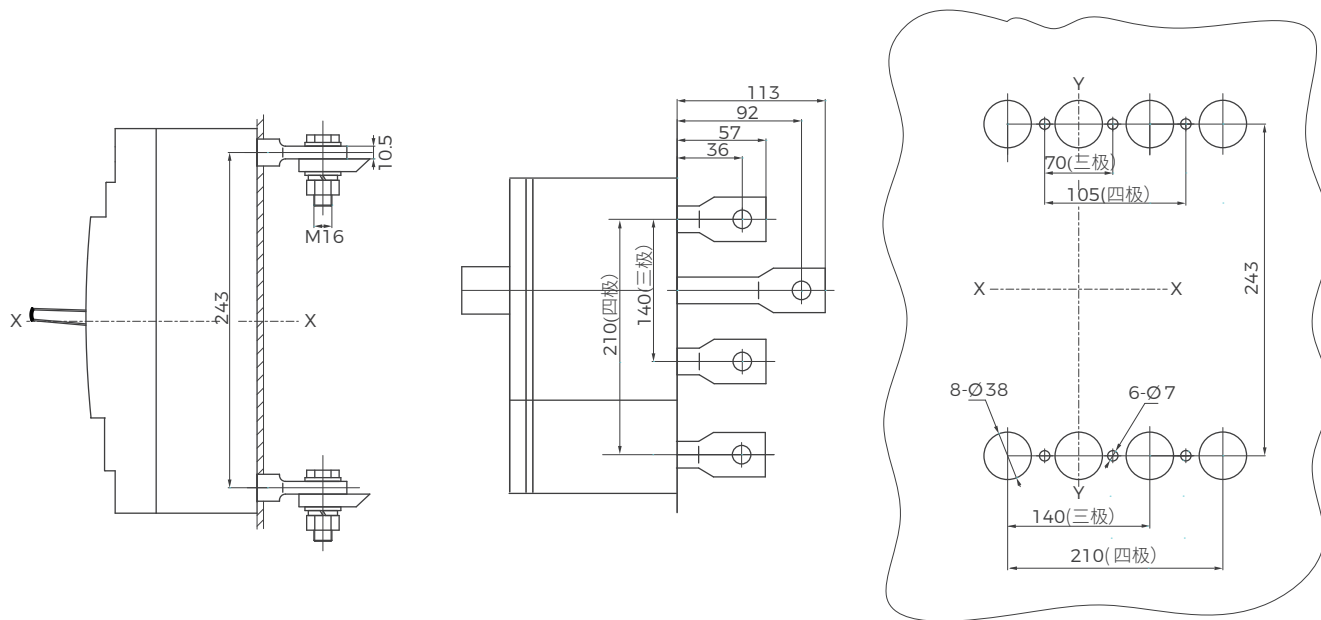
BM3E-630M/H 塑壳断路器板后接线
