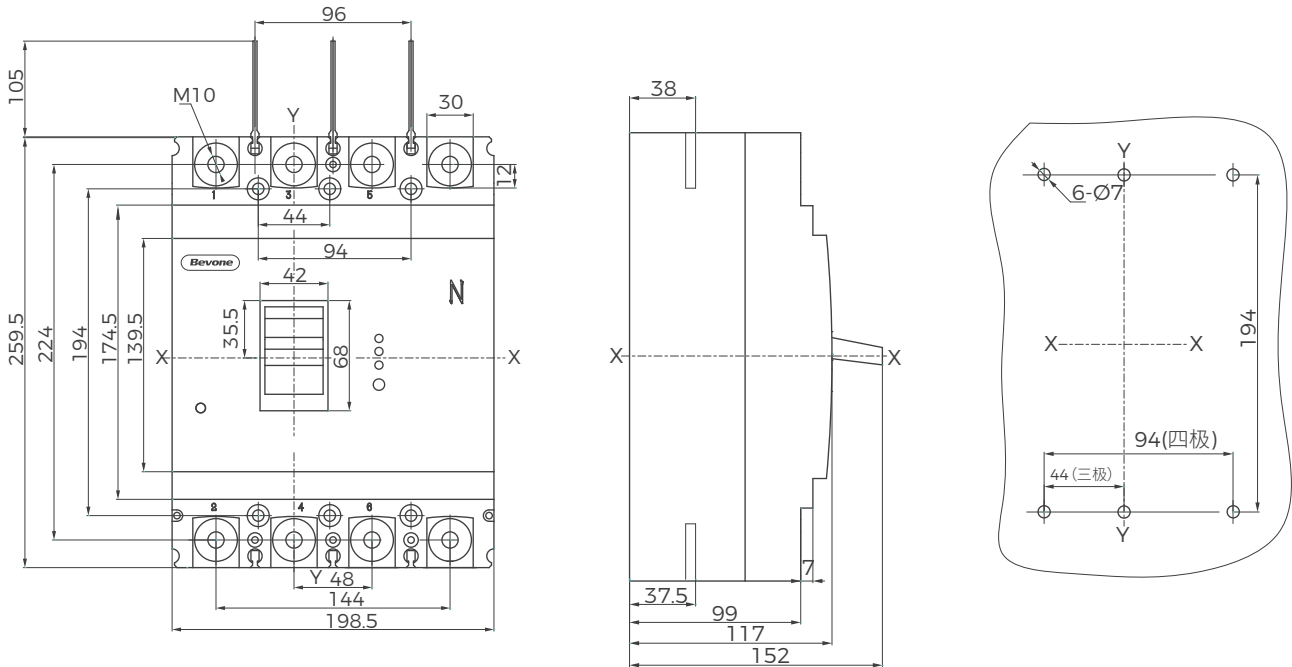
BM3L-400 (四极)
