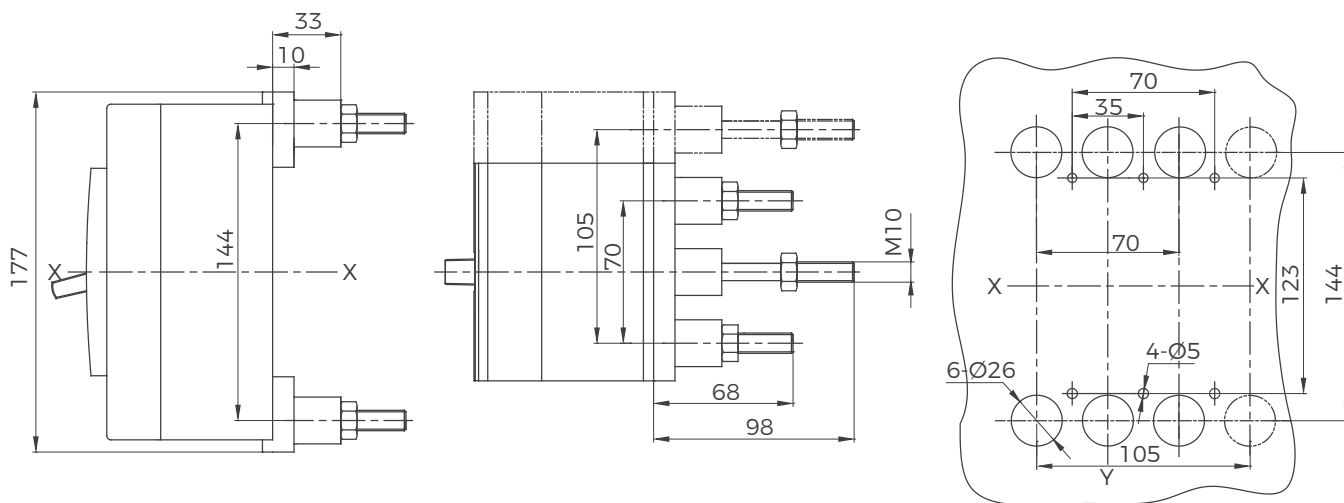
BM3-250 (C、F、L、N、M、S、H) 插入式板后接线 (三极、四极)
