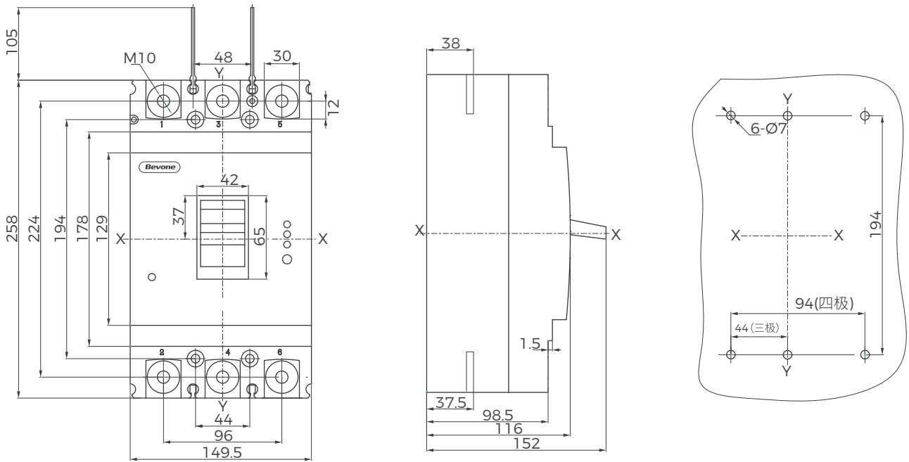
BM3L-400 (三极)
