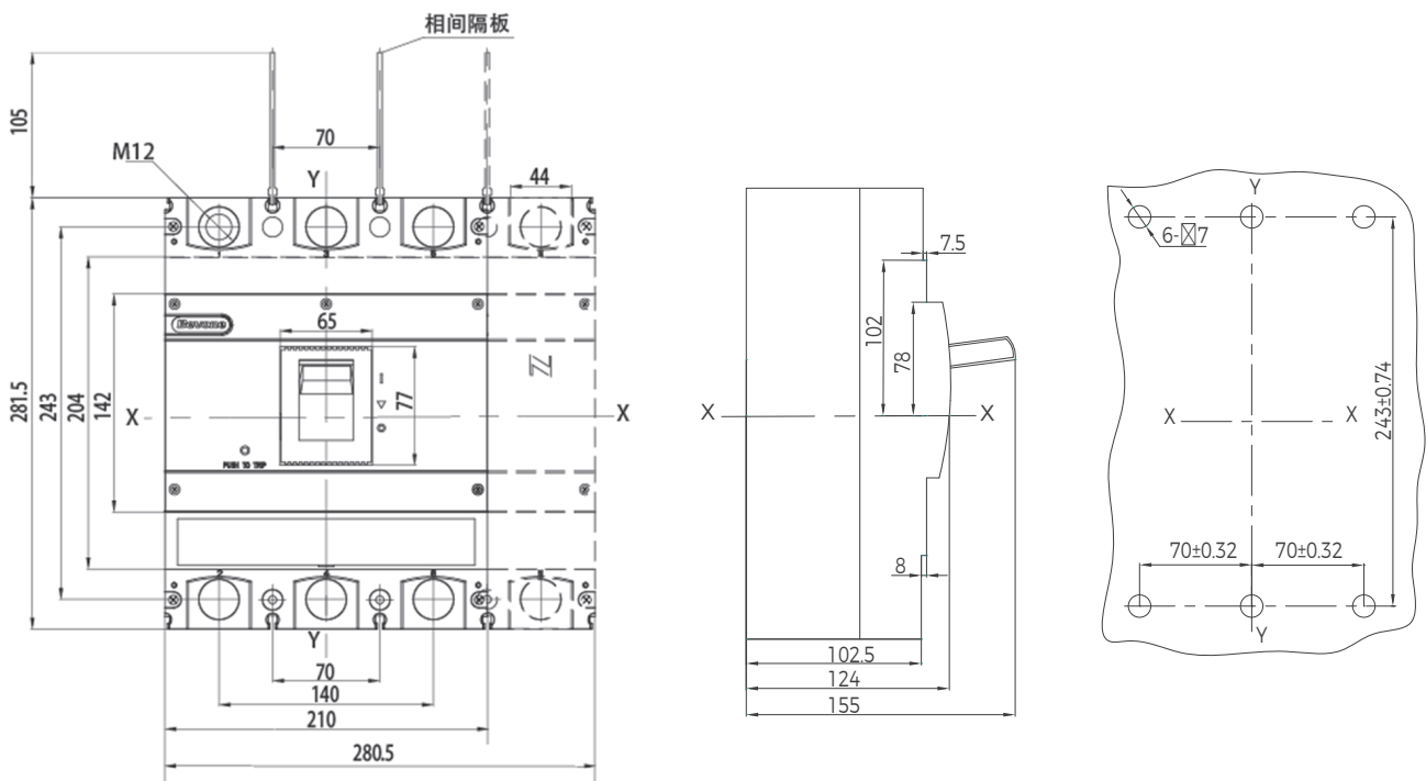
BM3E-630M/H 塑壳断路器板前接线
