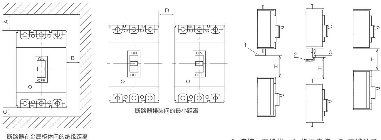
BM3 系列塑料外壳式断路器安全距离 (mm)
