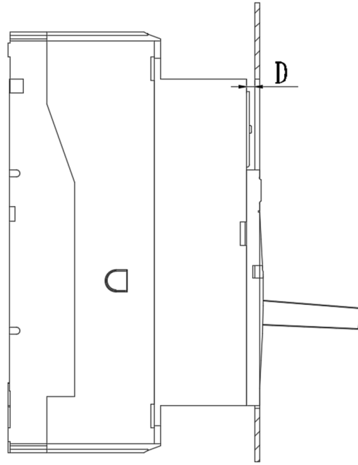
断路器与屏前最小距离 D=0
