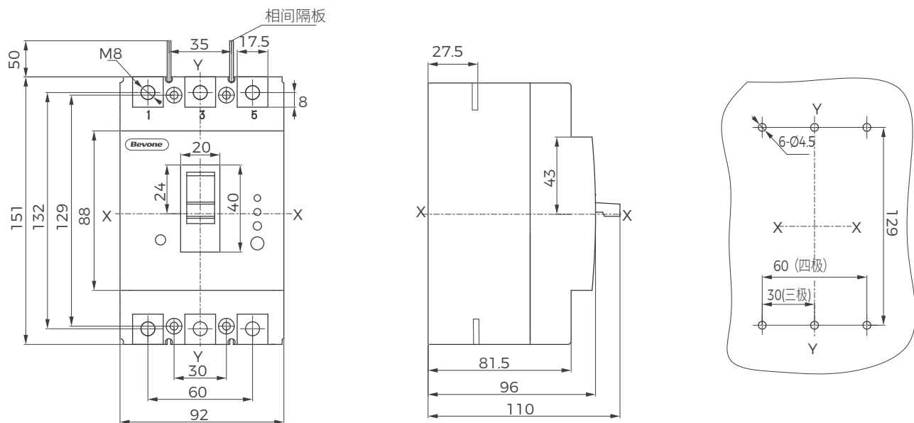
BM3L-125 (三极)
