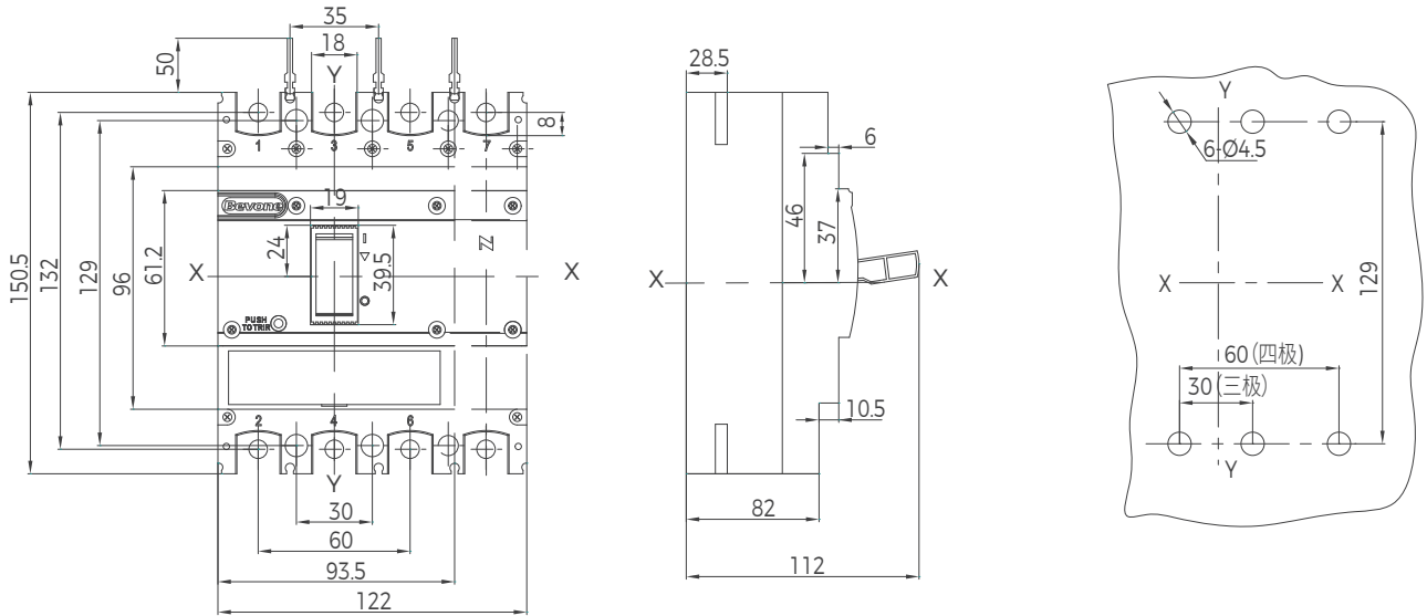
BM3E-125M/H 塑壳断路器板前接线
