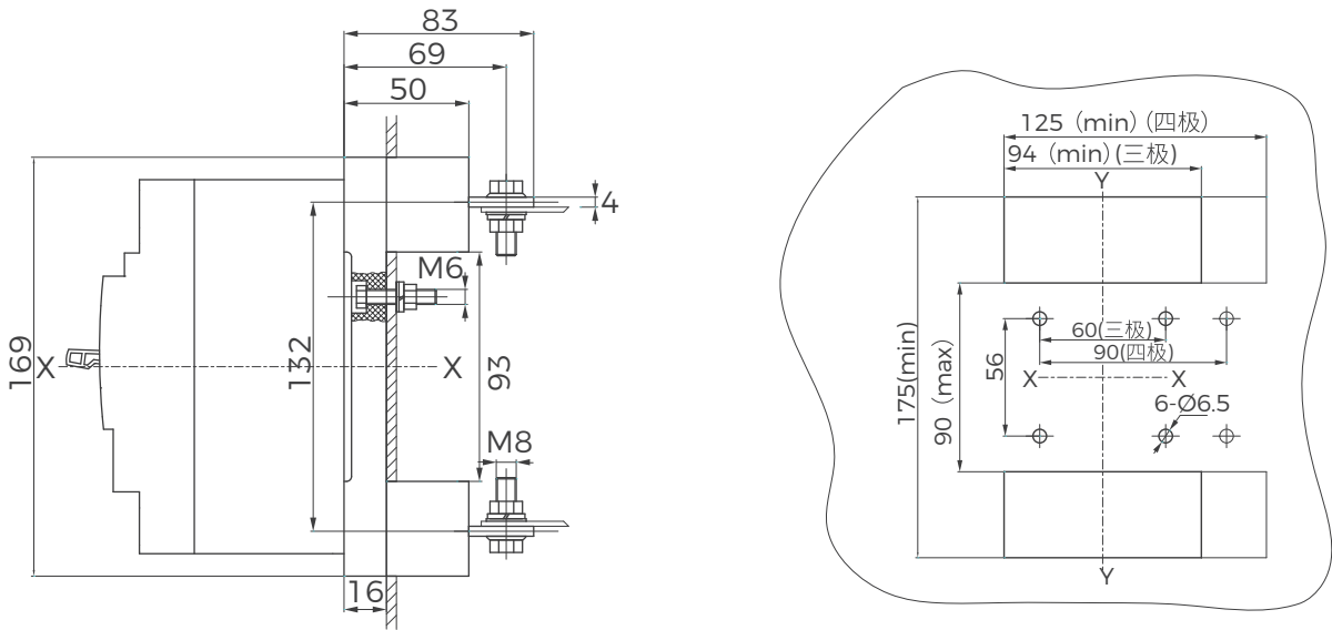
BM3E-125M/H 塑壳断路器插入式板后接线
