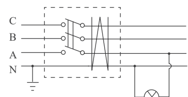
正确接线
