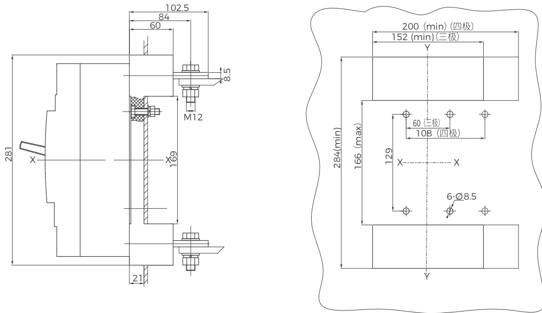
BM3E-400M/H 塑壳断路器插入式板后接线
