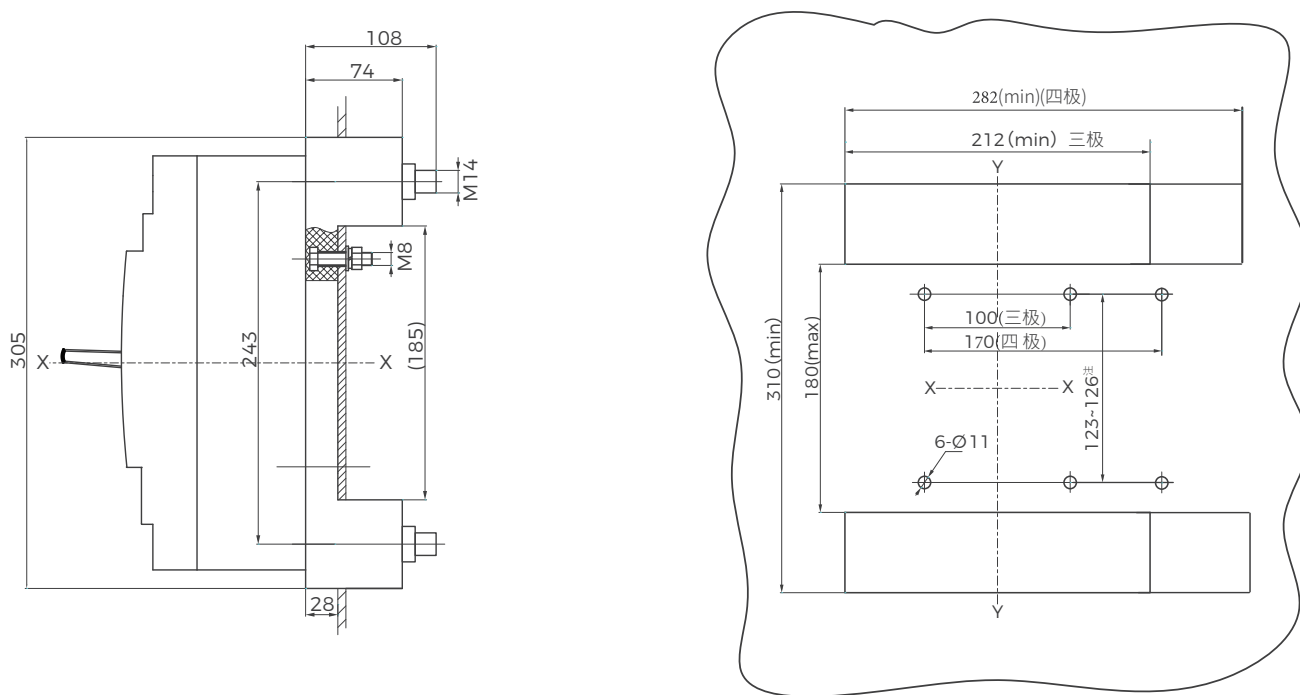
BM3E-630M/H 塑壳断路器插入式板后接线
