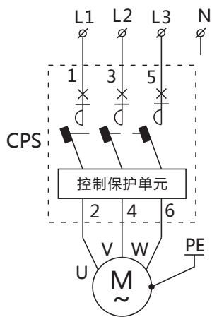
三相电动机连接电路图
