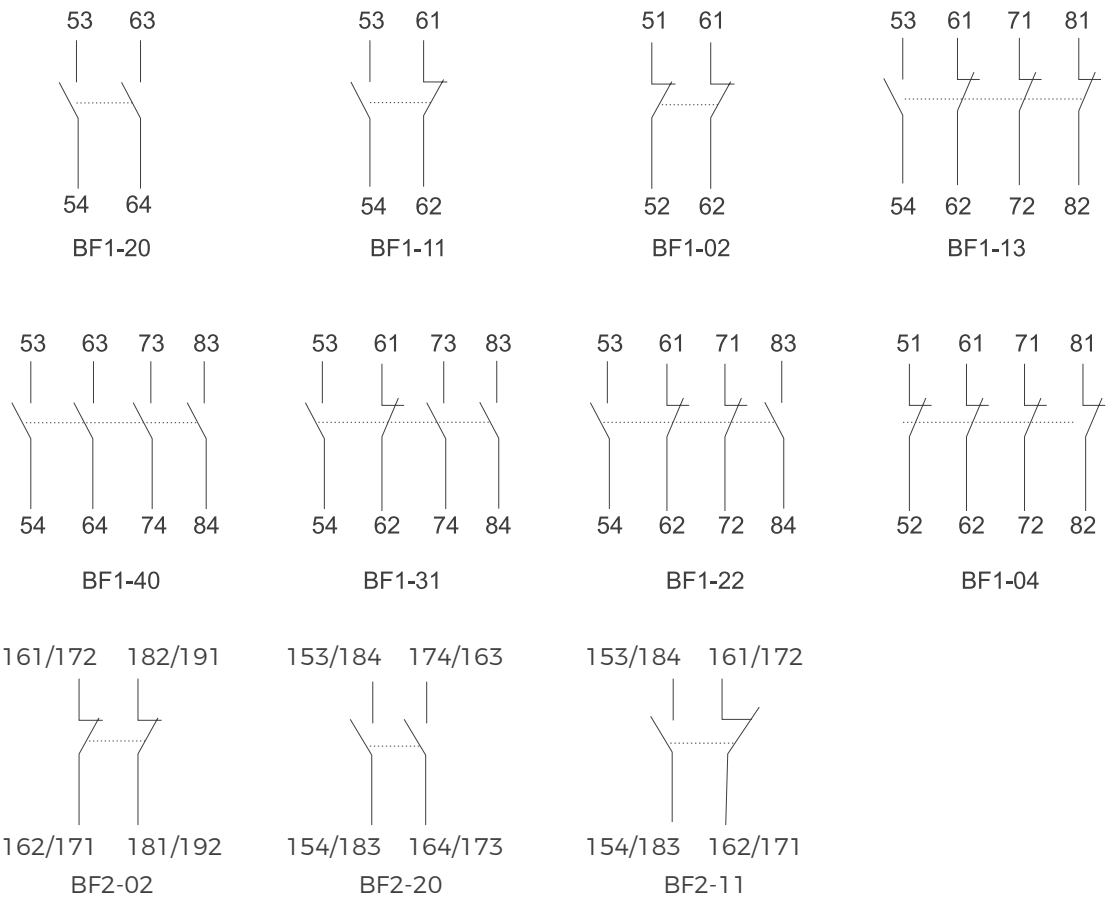
辅助触头组接线图
