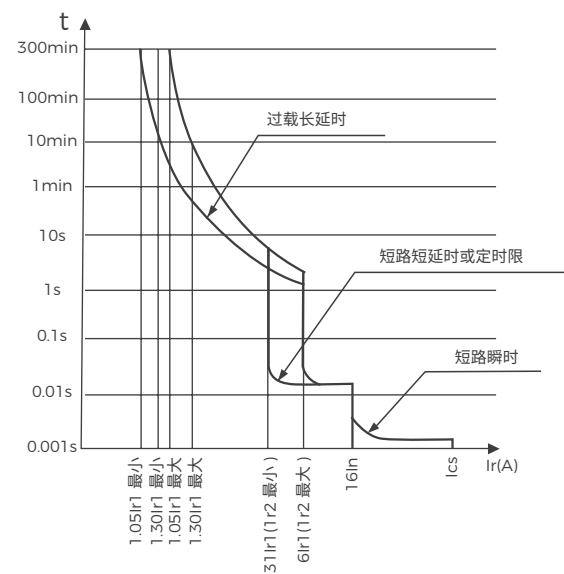
BK2 配电保护时间电流特性
