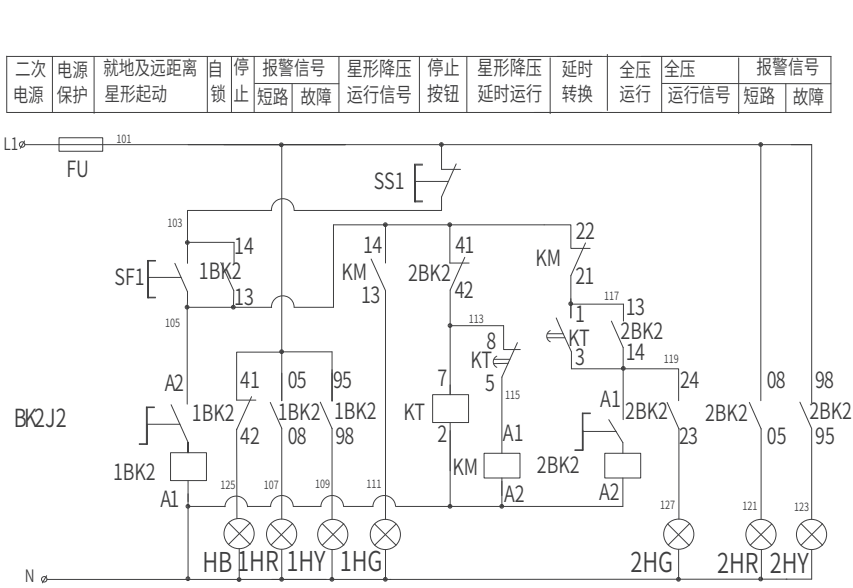
BK2J2 星三角（06M）接线原理图（45kW 以上）
