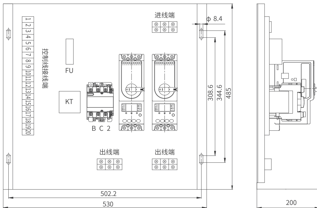
BK2J2-125 外形及安装尺寸
