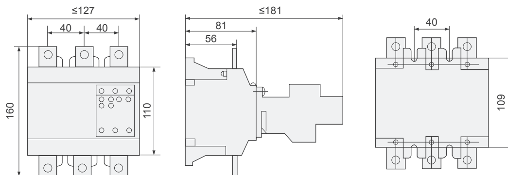
BR2-200 外形与安装尺寸
