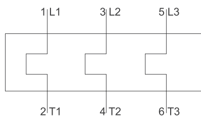
主电路
