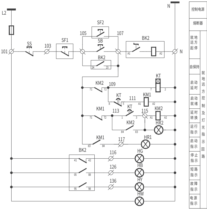
BK2J 星三角（06M）接线原理图
