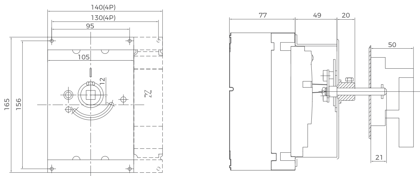
图 11 BM5-160/250 手操开孔尺寸
