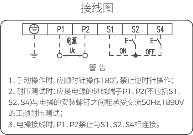
图 8 电操接线图
