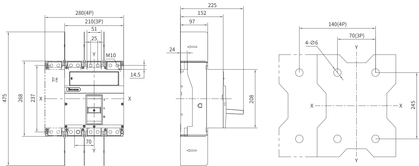
BM5-1600 外形尺寸 (3P/4P)
