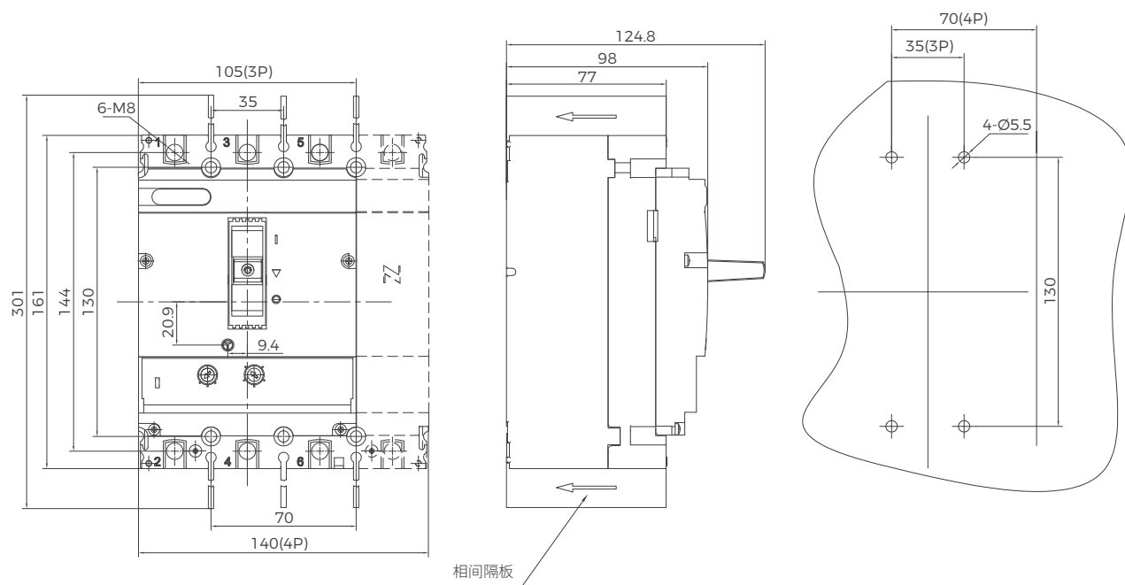
BM5-160(L、M、H) 外形尺寸 (3P/4P)
