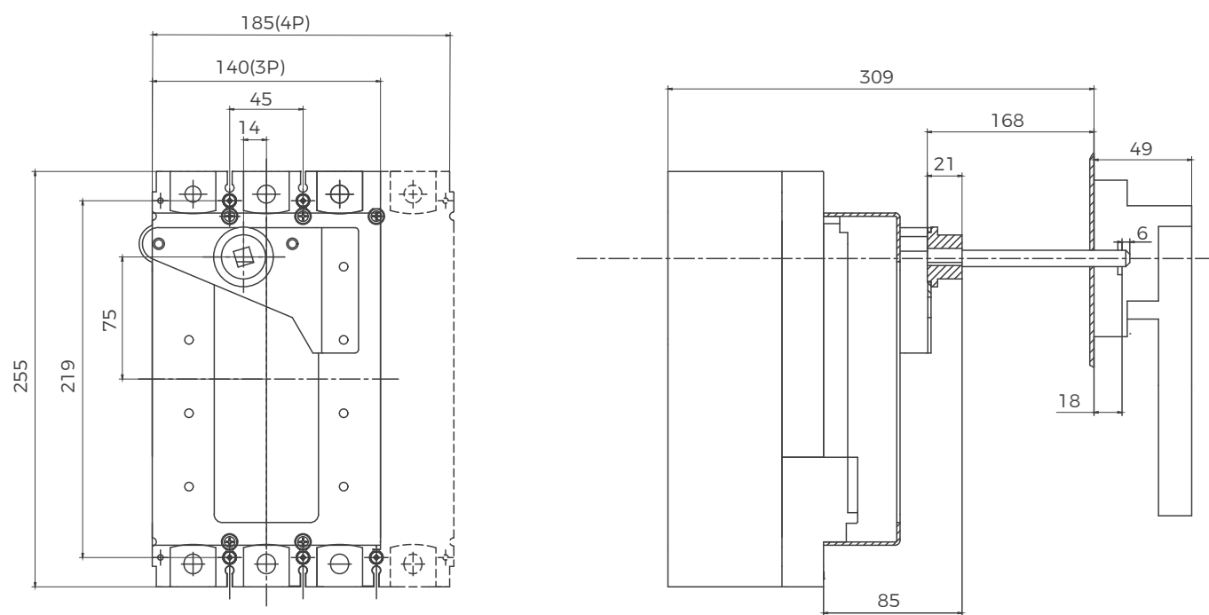
图 12 BM5-400/630 手操开孔尺寸
