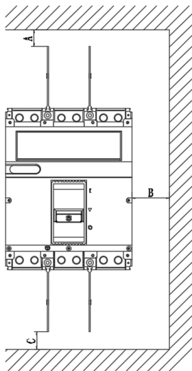
断路器之间最小距离
