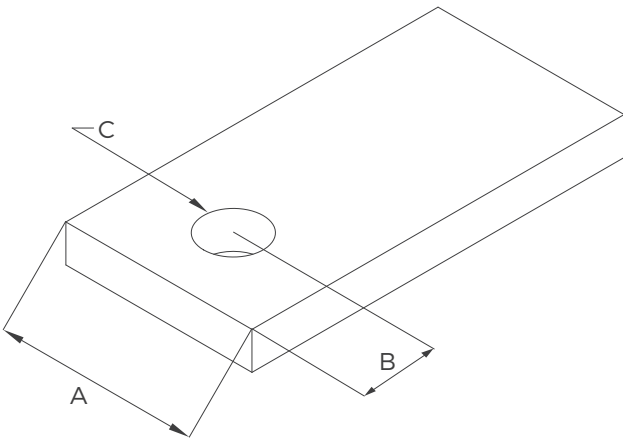
联接排尺寸
