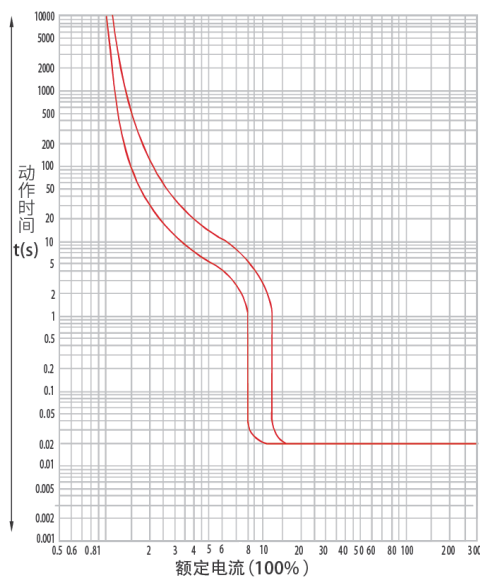
时间/特性曲线
