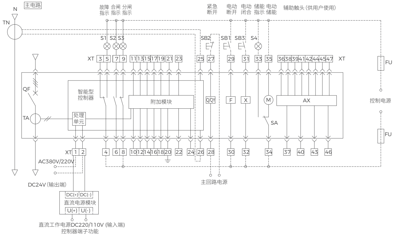
工作原理图 BW1-1600 的二次接线图
