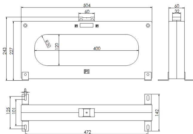
图 26-2 ZCT1-400 互感器
