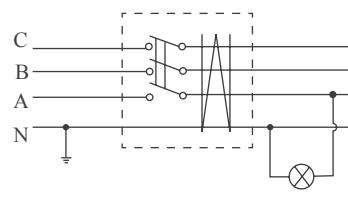
正确接线
