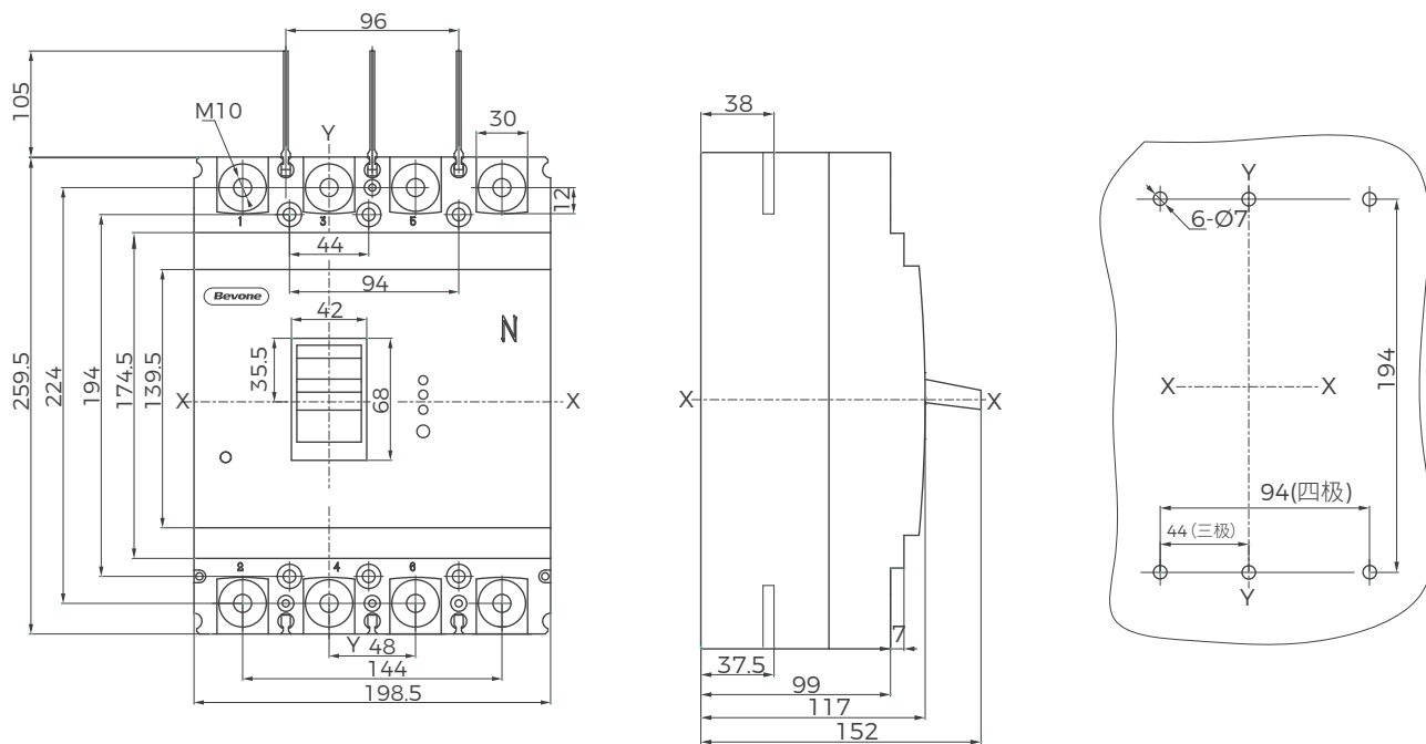
BM3L-400 (四极)
