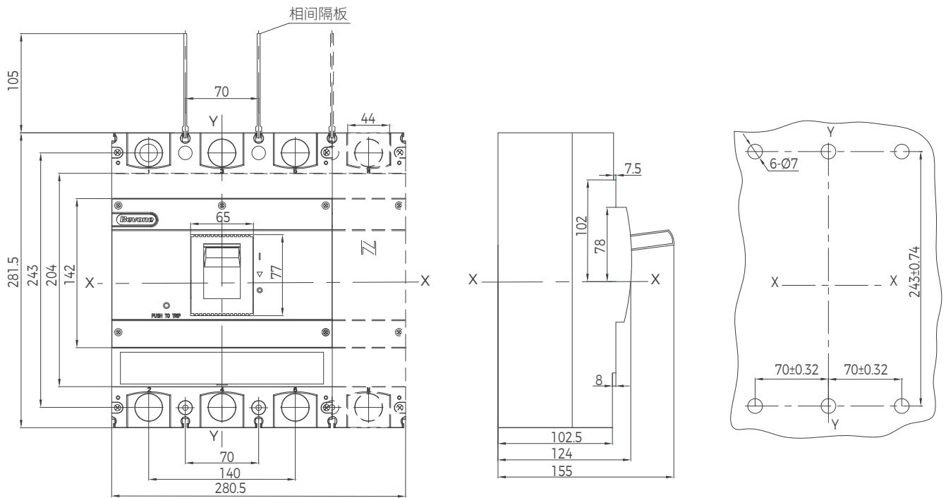
BM3E-800M/H 塑壳断路器板前接线
