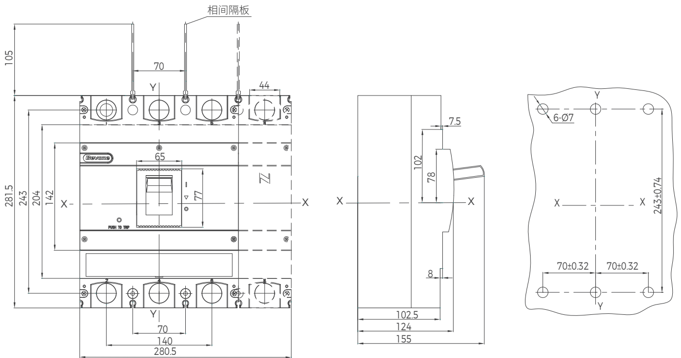
BM3E-630M/H 塑壳断路器板前接线
