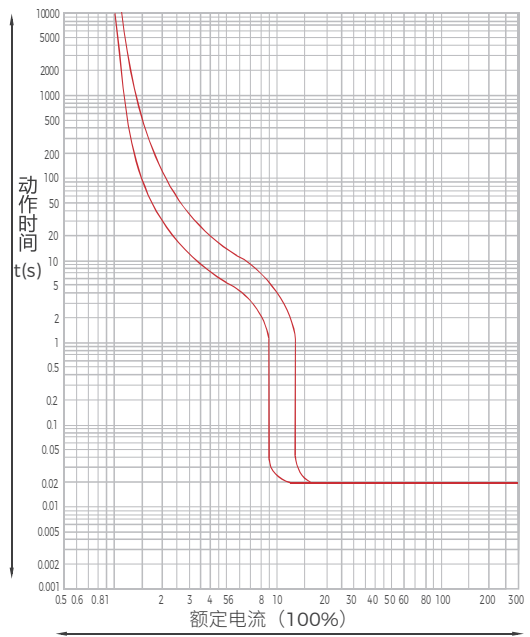
时间/特性曲线
