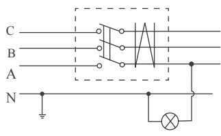
错误接线
