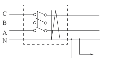
错误接线
