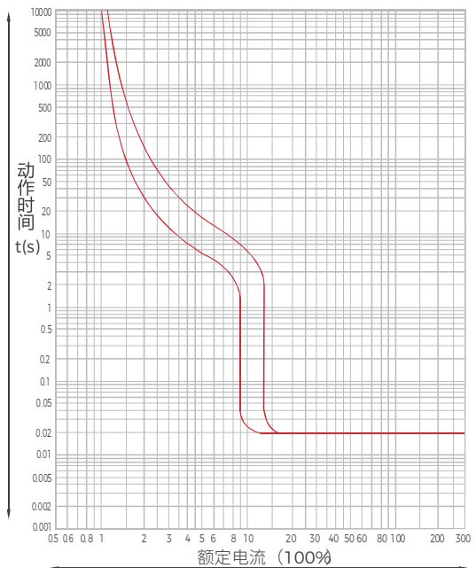
时间/特性曲线
