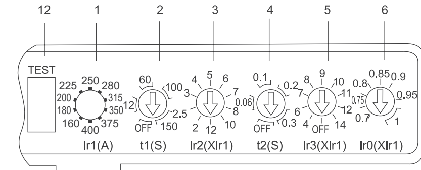
BM3E-400, In=400A 电子式脱扣器
