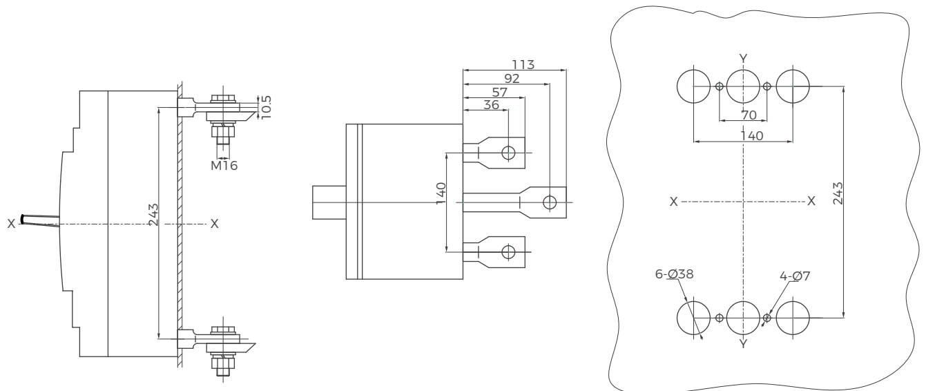
BM3E-800M/H 塑壳断路器板后接线
