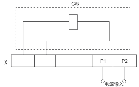
外挂欠电压脱扣器模块接线图 (虚框内为断路器内部附件接线图)
