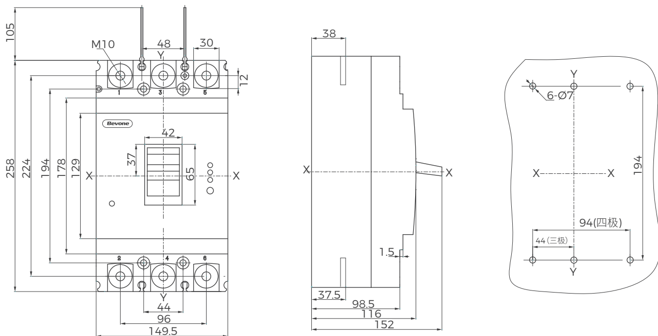
BM3L-400 (三极)
