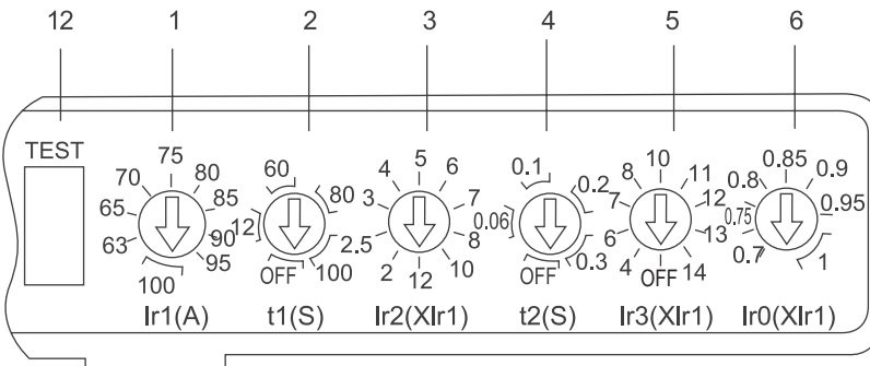
BM30E-100, In=100A 电子式脱扣器
