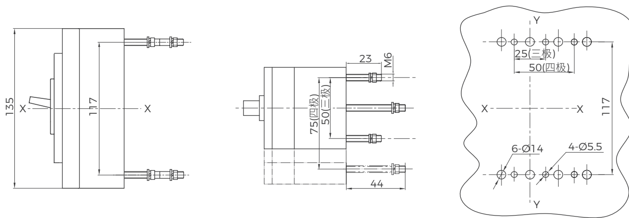
BM30-63 (L、M) 板后接线 (三极、四极)
