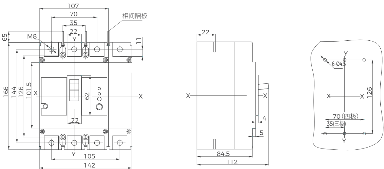
BM30L-250 (三极、四极)
