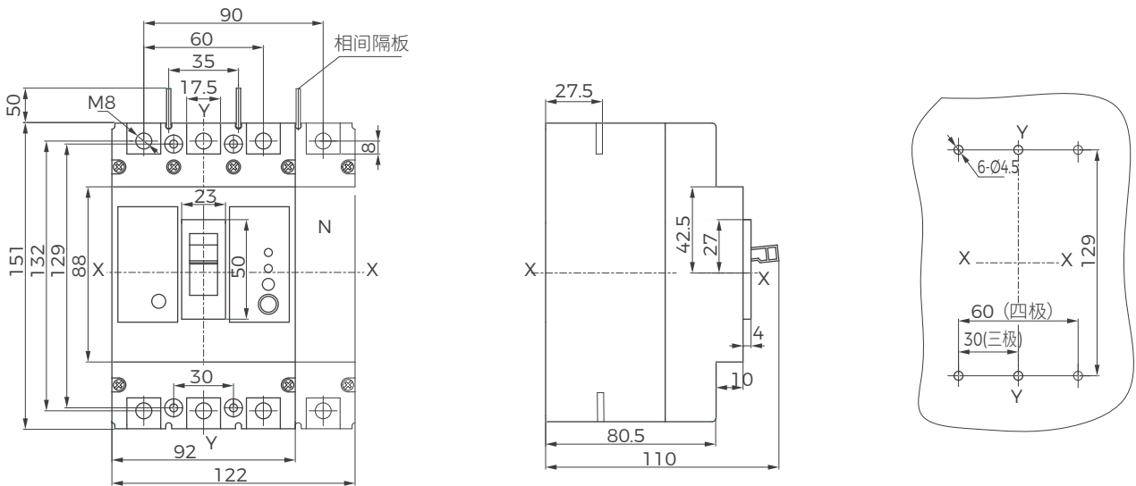
BM30L-125 (三极、四极)
