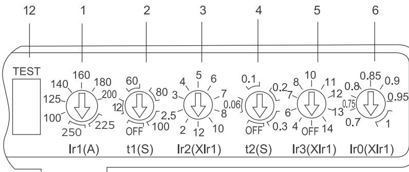
BM30E-250, In=250A 电子式脱扣器
