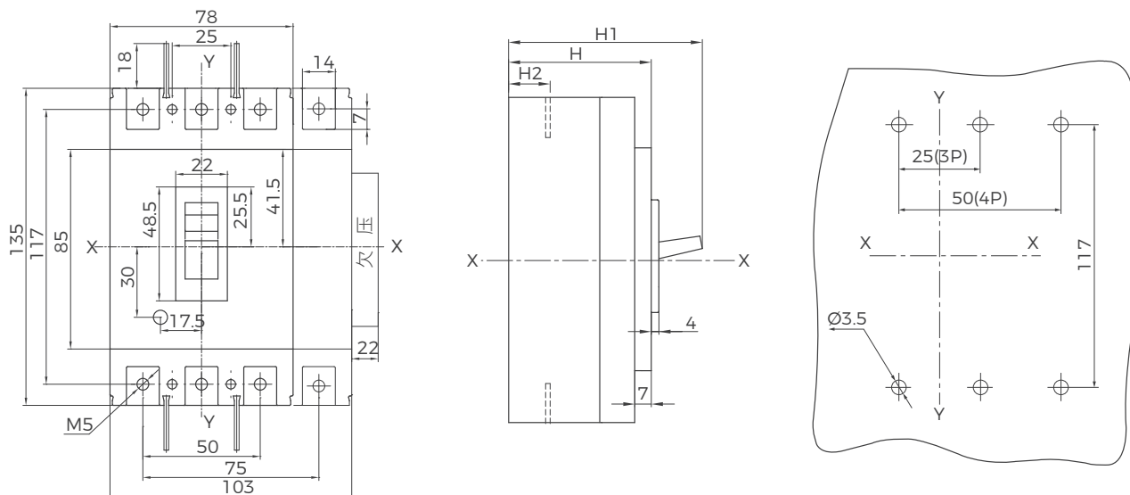
BM30-63 (L、M) 板前接线 (三极、四极)
